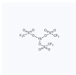
1093017 CAS: 54761-04-5
