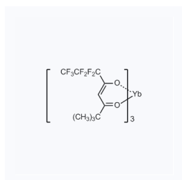
1024230 CAS: 18323-96-1
