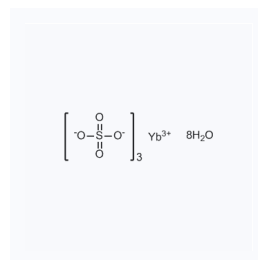
1182223 CAS: 10034-98-7
