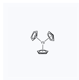
1181152 CAS: 1295-20-1
