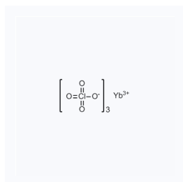
1182221 CAS: 13498-08-3
