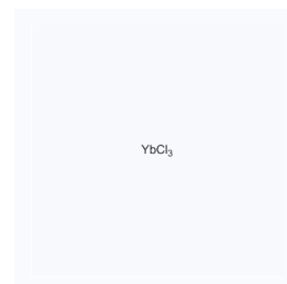
1156387 CAS: 10361-91-8
