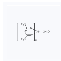
1181138 CAS: 81849-60-7
