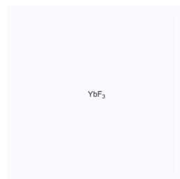
1182215 CAS: 13760-80-0
