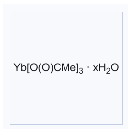
1182195 CAS: 15280-58-7
