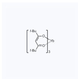
1182192 CAS: 15492-52-1
