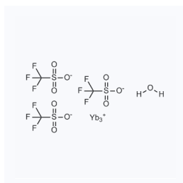
1169657 CAS: 252976-51-5
