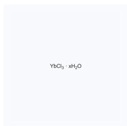
1182214 CAS: 19423-87-1
