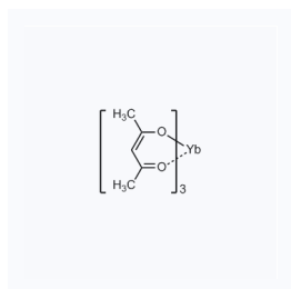
1182197 CAS: 14284-98-1
