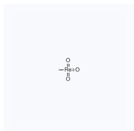
1182398 CAS: 70197-13-6
