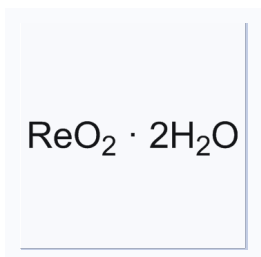
1182428 CAS: 12036-09-8
