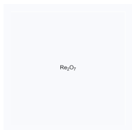
1182429 CAS: 1314-68-7
