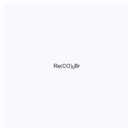
1176749 CAS: 14220-21-4
