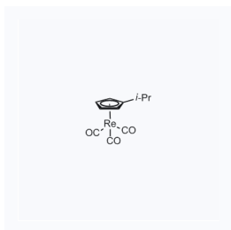
1182425 CAS: 126250-68-8
