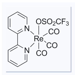
1182433 CAS: 97170-94-0
