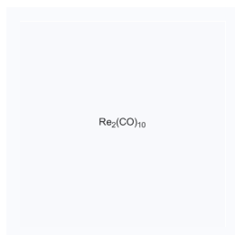
1176696 CAS: 14285-68-8
