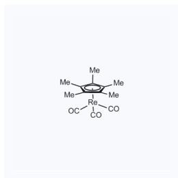
1182423 CAS: 12130-88-0
