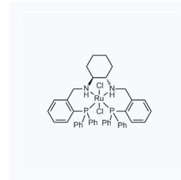
1152678 CAS: 302924-37-4
