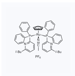
1152725 CAS: 776230-17-2
