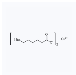
1181666 现货 CAS: 50315-14-5
