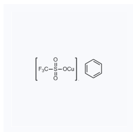
1155945 CAS: 42152-46-5
