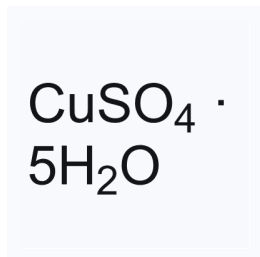
1042960 现货 CAS: 7758-99-8
