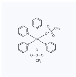
1171161 CAS: 113110-58-0
