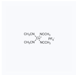
1105913 现货 CAS: 64443-05-6
