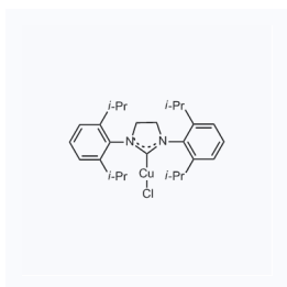
1202688 CAS: 915395-52-7
