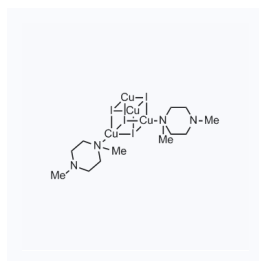
1181650 CAS: 1401708-91-5
