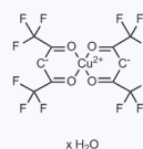
1022506 CAS: 155640-85-0
