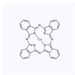
1177028 CAS: 147-14-8
