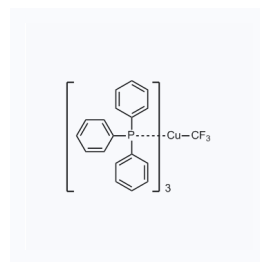
1177306 CAS: 325810-07-9
