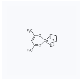
1155947 现货 CAS: 86233-74-1
