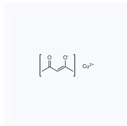
1155938 现货 CAS: 13395-16-9
