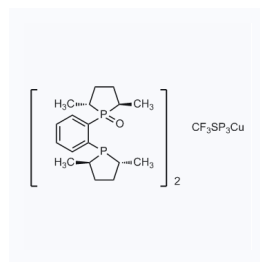
1177532 CAS: 874013-62-4
