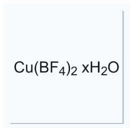
1181678 现货 CAS: 207121-39-9
