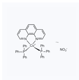
1105902 CAS: 33989-10-5
