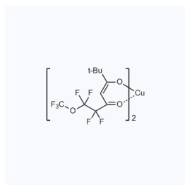
1043975 CAS: 80289-21-0
