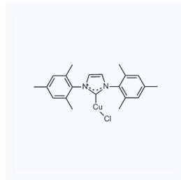
1045370 现货 CAS: 873779-78-3
