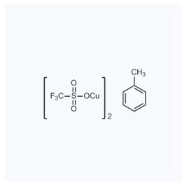
1105909 现货 CAS: 48209-28-5
