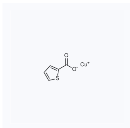
1091826 现货 CAS: 68986-76-5
