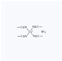
1155939 现货 CAS: 15418-29-8
