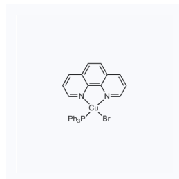
1158416 现货 CAS: 25753-84-8
