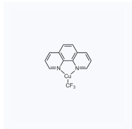
1155937 现货 CAS: 1300746-79-5
