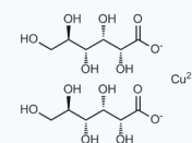
1034692 CAS: 527-09-3
