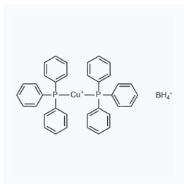
1156310 CAS: 16903-61-0
