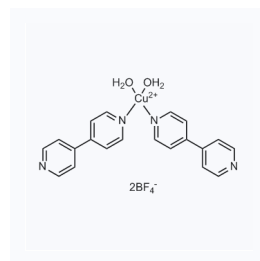
1155975 CAS: 854623-98-6
