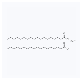
1066274 现货 CAS: 660-60-6
