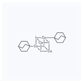
1181635 CAS: 928170-42-7
