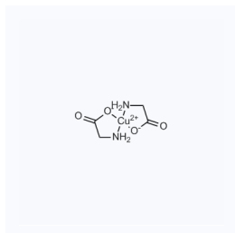
1069359 现货 CAS: 13479-54-4
