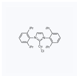
1156314 现货 CAS: 578743-87-0
