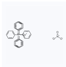
1105789 CAS: 106678-35-7
