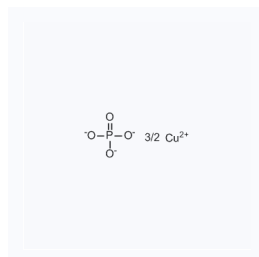
1213452 现货 CAS: 7798-23-4
