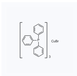
1022623 现货 CAS: 15709-74-7
