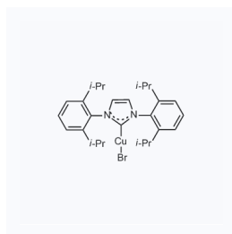
1202683 CAS: 915395-54-9
