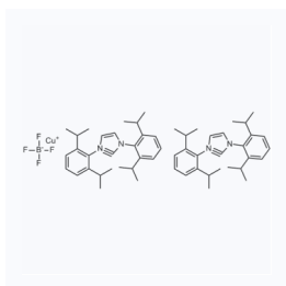
1045660 CAS: 886061-48-9
