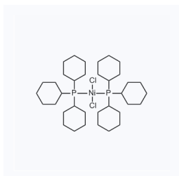
1105881 现货 CAS: 19999-87-2
