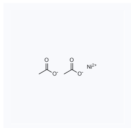
1155165 现货 CAS: 373-02-4
