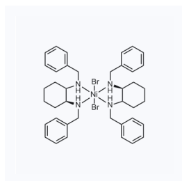
1124017 CAS: 941321-22-8
