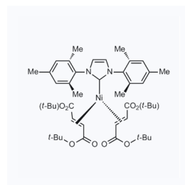
1181411 CAS: 2091838-72-9
