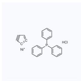
1029389 CAS: 31904-79-7
