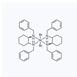
1119452 CAS: 941321-23-9
