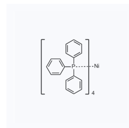
1112938 CAS: 15133-82-1
