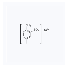
1156016 CAS: 375387-13-6
