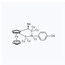
1181324 CAS: 2049086-35-1
