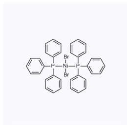
1156212 现货 CAS: 14126-37-5
