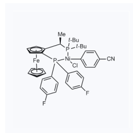
1181326 CAS: 2049086-37-3
