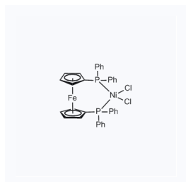
1039540 现货 CAS: 67292-34-6
