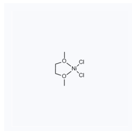
1112958 现货 CAS: 29046-78-4
