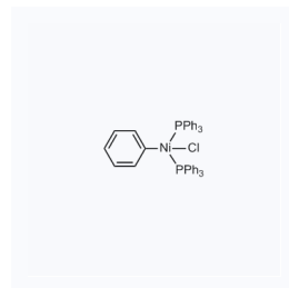
1181463 CAS: 33571-43-6
