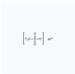
1156220 现货 CAS: 60871-84-3
