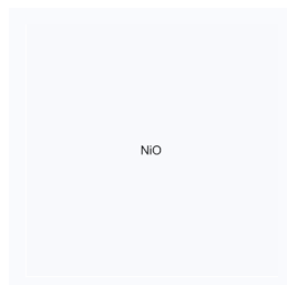
1181612 现货 CAS: 1313-99-1
