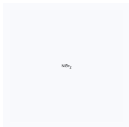
1156271 现货 CAS: 13462-88-9
