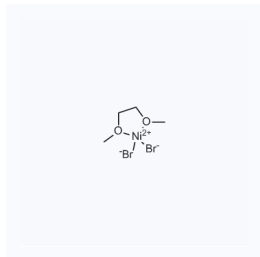
1170447 现货 CAS: 28923-39-9
