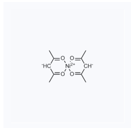
1029628 现货 CAS: 3264-82-2
