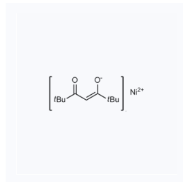
1157046 现货 CAS: 14481-08-4
