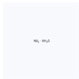
1181592 CAS: 7790-34-3
