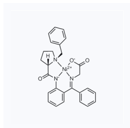
1060556 现货 CAS: 96293-19-5
