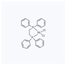
1021728 现货 CAS: 14647-23-5
