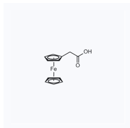
1019264 现货 CAS: 1287-16-7
