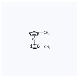
1176618 现货 CAS: 1291-47-0
