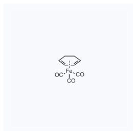
1177377 现货 CAS: 12152-72-6
