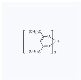
1021949 现货 CAS: 14876-47-2
