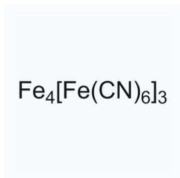
1097187 现货 CAS: 14038-43-8
