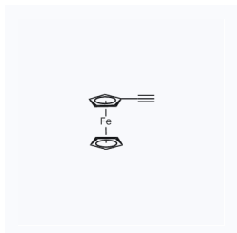
1019127 现货 CAS: 1271-47-2
