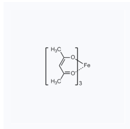
1181814 现货 CAS: 14024-18-1
