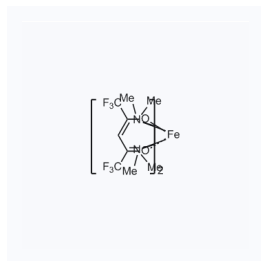
1181805 CAS: 73450-43-8
