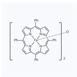
1176551 CAS: 12582-61-5
