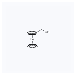
1106757 现货 CAS: 1273-86-5
