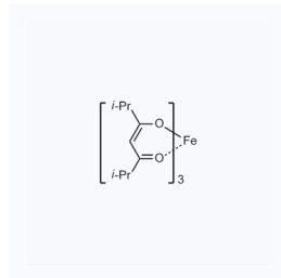
1181799 现货 CAS: 24444-72-2
