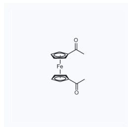
1019164 现货 CAS: 1273-94-5
