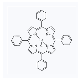
1099568 CAS: 16456-81-8
