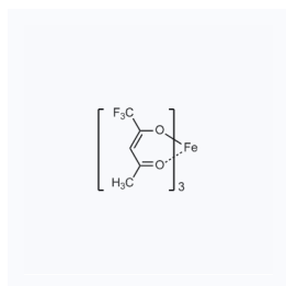
1021613 CAS: 14526-22-8
