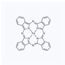
1176627 CAS: 132-16-1
