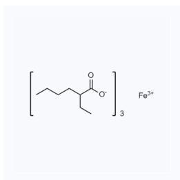
1177392 CAS: 7321-53-1
