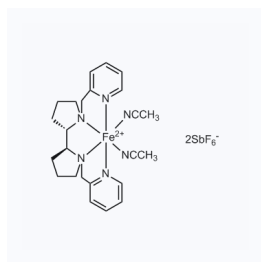
1181809 CAS: 959395-10-9
