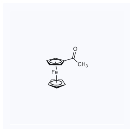
1070174 现货 CAS: 1271-55-2
