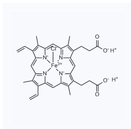
1085483 现货 CAS: 16009-13-5
