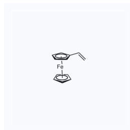
1176593 现货 CAS: 1271-51-8
