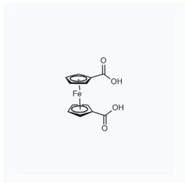
1176620 现货 CAS: 1293-87-4
