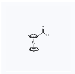
1113763 现货 CAS: 12093-10-6
