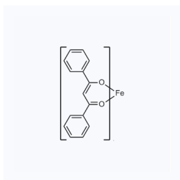
1156118 CAS: 14405-49-3
