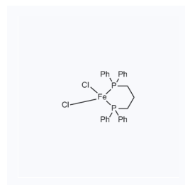
1181812 CAS: 106245-43-6
