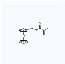
1156110 现货 CAS: 31566-61-7
