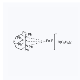
1181877 CAS: 1318882-57-3
