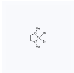
1181818 现货 CAS: 99611-53-7
