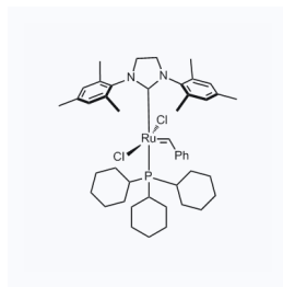
1089763 现货 CAS: 246047-72-3
