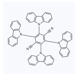
1157329 CAS: 1416881-53-2
