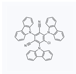
1176294 CAS: 1469704-61-7
