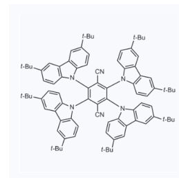
1175929 CAS: 2153433-46-4
