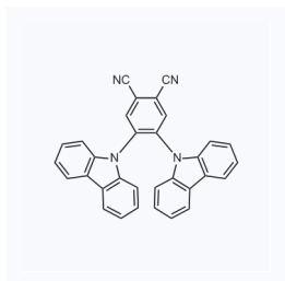
1176317 CAS: 1416881-50-9
