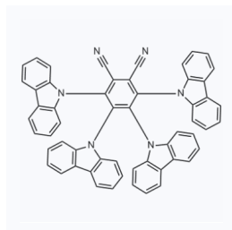
1176318 CAS: 1416881-51-0
