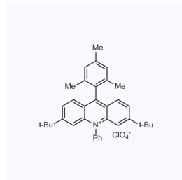
1175833 现货 CAS: 2377107-96-3
