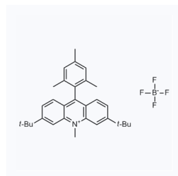
1176227 CAS: 2054779-48-3
