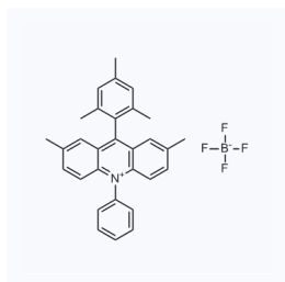
1176174 CAS: 1621020-00-5
