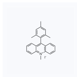
1176245 CAS: 930097-17-9
