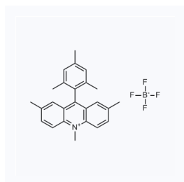
1176208 CAS: 1621019-97-3
