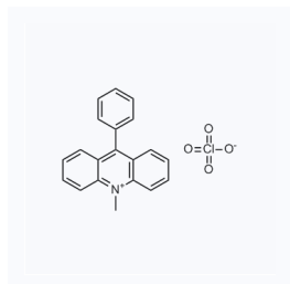
1176248 现货 CAS: 36519-61-6
