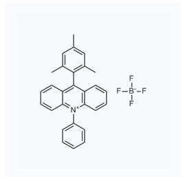
1169635 现货 CAS: 1621019-96-2
