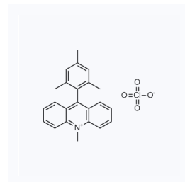
1174029 现货 CAS: 674783-97-2
