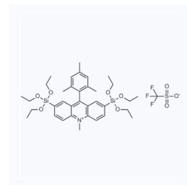
1176296 CAS: 1261648-50-3
