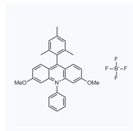
1176214 CAS: 1965330-57-7
