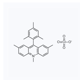
1176209 CAS: 1216909-33-9
