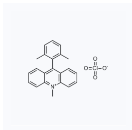
1176246 现货 CAS: 1276539-32-2
