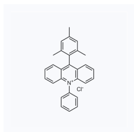
1176190 CAS: 2088856-21-5
