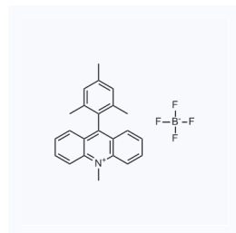
1176172 现货 CAS: 1442433-71-7
