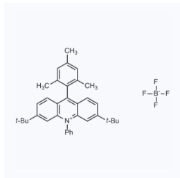
1175900 现货 CAS: 1810004-87-5
