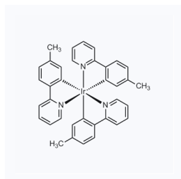
1181214 现货 CAS: 149005-33-4
