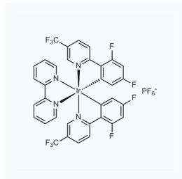
1153401 现货 CAS: 1092775-62-6
