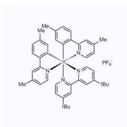
1153436 CAS: 1607469-49-7
