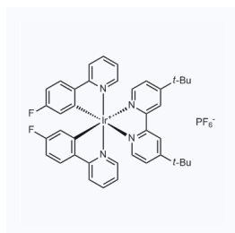
1180589 CAS: 1449110-90-0
