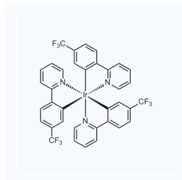
1153446 现货 CAS: 500295-52-3
