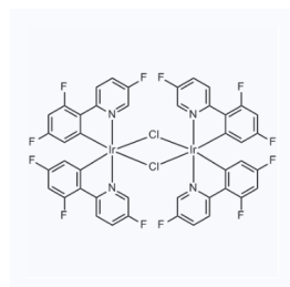
1181219 CAS: 849723-04-2
