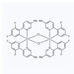
1153573 CAS: 1335047-33-0
