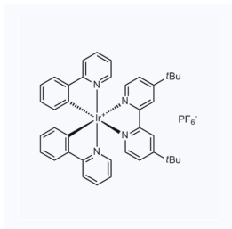
1153235 现货 CAS: 676525-77-2
