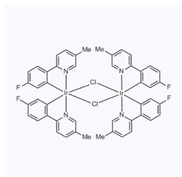
1153565 现货 CAS: 808142-89-4
