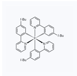
1181196 CAS: 359014-76-9
