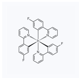
1153490 CAS: 370878-69-6
