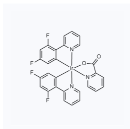
1031216 现货 CAS: 376367-93-0
