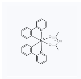
1030018 现货 CAS: 337526-85-9
