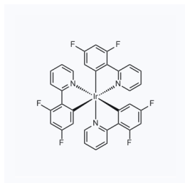
1153402 现货 CAS: 387859-70-3
