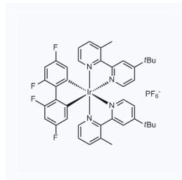
1153495 现货 CAS: 1335047-34-1
