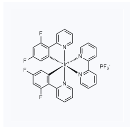
1158390 现货 CAS: 864163-80-4
