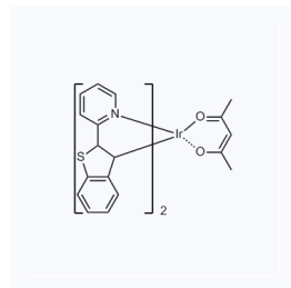
1181202 CAS: 343978-79-0
