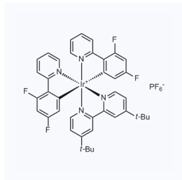
1153492 现货 CAS: 1072067-44-7
