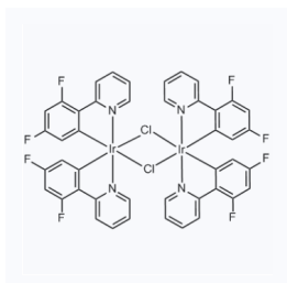
1153500 现货 CAS: 562824-27-5
