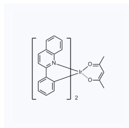
1181204 现货 CAS: 1173886-71-9
