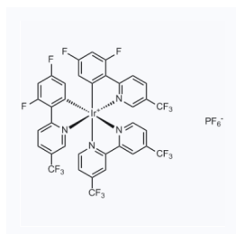
1181216 CAS: 2030437-90-0
