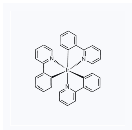
1047180 现货 CAS: 94928-86-6
