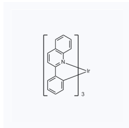
1181212 CAS: 911142-72-8
