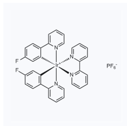
1180588 现货 CAS: 1580547-45-0
