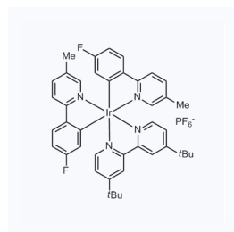
1153548 CAS: 808142-88-3
