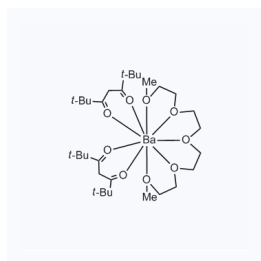
1182636 CAS: 136629-60-2
