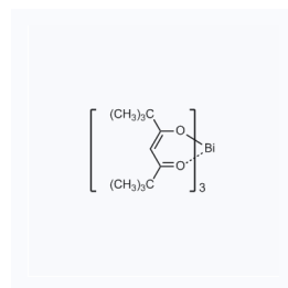
1177483 CAS: 142617-53-6
