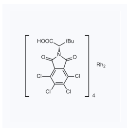
1034319 CAS: 515876-71-8
