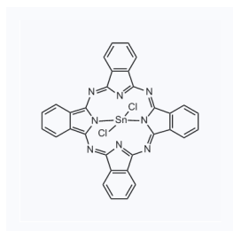
1182191 CAS: 18253-54-8
