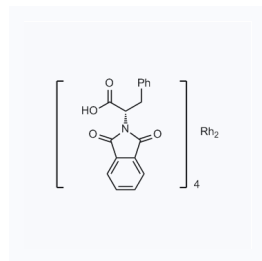
1019639 CAS: 131219-55-1
