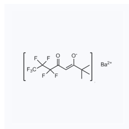
1157346 CAS: 36885-31-1
