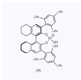
1161764 现货 CAS: 929294-27-9
