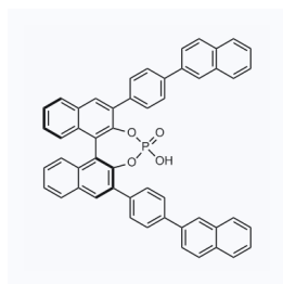
1162575 CAS: 871130-15-3
