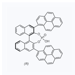
1161767 CAS: 2270966-57-7
