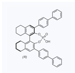
1164014 现货 CAS: 861909-35-5
