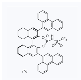
1163553 现货 CAS: 1181834-74-1
