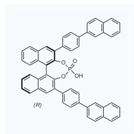
1162120 CAS: 699006-55-8
