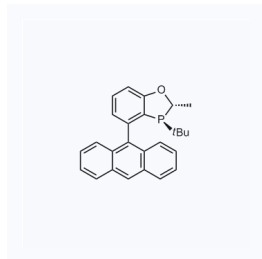
1161717 现货 CAS: 1884594-02-8
