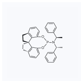
1107971 现货 CAS: 500997-69-3
