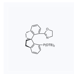
1131510 现货 CAS: 1040274-18-7
