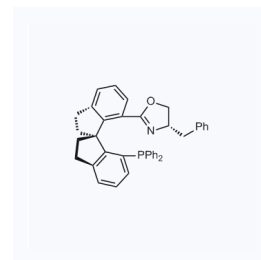
1108103 现货 CAS: 913829-88-6
