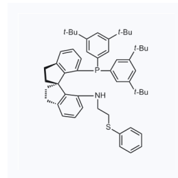
1178760 CAS: 1809609-38-8
