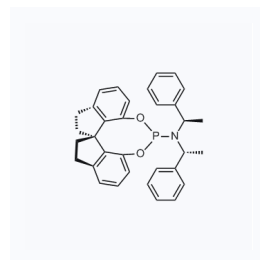
1156706 现货 CAS: 500997-70-6
