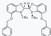
1184274 CAS: 1994323-92-0
