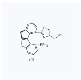
1161869 现货 CAS: 2074610-05-0
