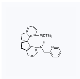
1161864 现货 CAS: 1415636-82-6
