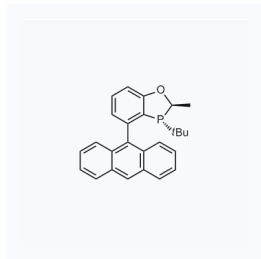
1161715 现货 CAS: 1477517-20-6
