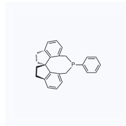
1108266 CAS: 885701-78-0
