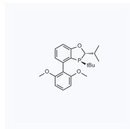
1105629 现货 CAS: 1477517-21-7
