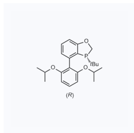
1161700 现货 CAS: 1338454-38-8
