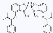
1184275 CAS: 2376521-83-2
