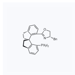
1131723 现货 CAS: 913829-90-0
