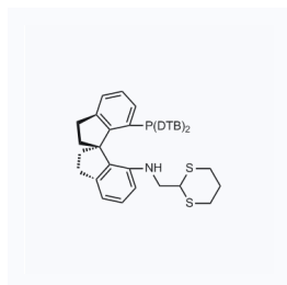
1130291 现货 CAS: 1809609-53-7
