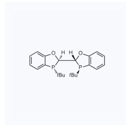
1159275 现货 CAS: 1610785-35-7
