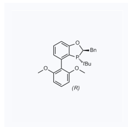
1162861 现货 CAS: 1884457-36-6
