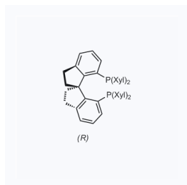
1133119 现货 CAS: 917377-75-4
