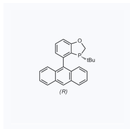
1090127 现货 CAS: 1456816-37-7
