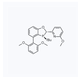
1161739 现货 CAS: 2003230-67-7
