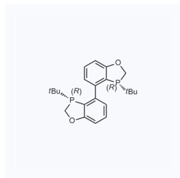
1162835 现货 CAS: 2214207-73-3
