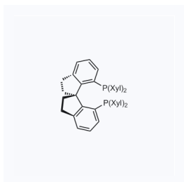
1107958 现货 CAS: 528521-89-3
