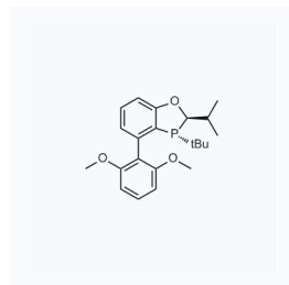
1105625 现货 CAS: 1477517-19-3
