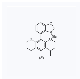
1162851 现货 CAS: 2351219-90-2
