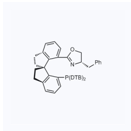
1107973 现货 CAS: 1040274-10-9
