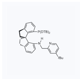
1161859 CAS: 1298133-38-6
