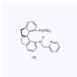
1130626 现货 CAS: 1298133-21-7
