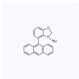
1090126 现货 CAS: 1268693-24-8
