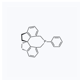
1108265 现货 CAS: 856407-37-9
