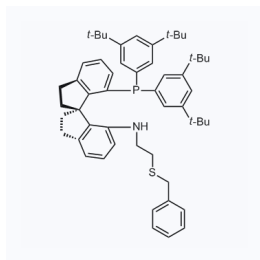
1178761 CAS: 1809609-52-6
