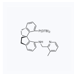
1205294 现货 CAS: 2177259-16-2
