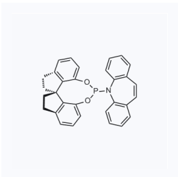
1208456 CAS: 1361055-07-3
