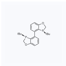
1161718 现货 CAS: 2207601-04-3
