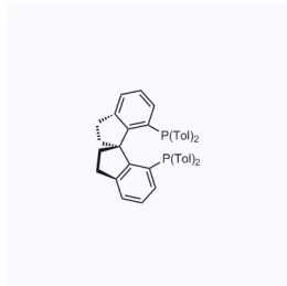
1133112 CAS: 817176-80-0
