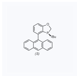
1090128 现货 CAS: 1807740-34-6
