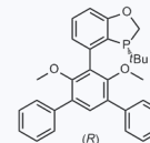
1162847 CAS: 2351219-89-9
