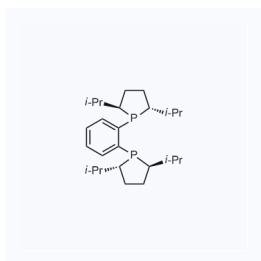
1176660 CAS: 136705-65-2
