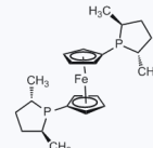
1174262 CAS: 162412-87-5
