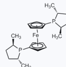
1174166 CAS: 540475-45-4
