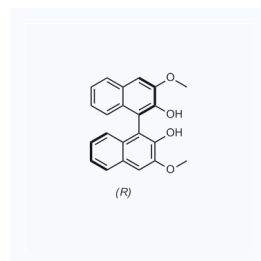
1167261 CAS: 63250-86-2
