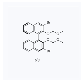
1157389 现货 CAS: 142010-87-5
