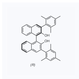
1157853 CAS: 394737-30-5
