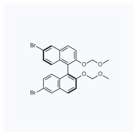
1105883 现货 CAS: 211560-97-3
