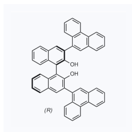
1159464 CAS: 1058734-56-7
