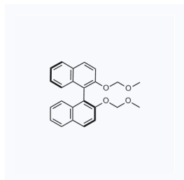
1021219 CAS: 142128-92-5
