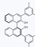
1157436 CAS: 435327-17-6
