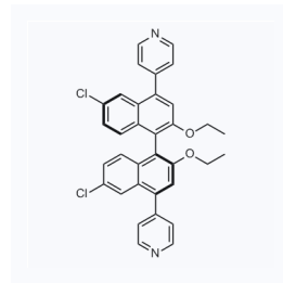
1158975 CAS: 431043-38-8
