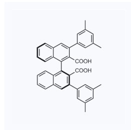
1167244 CAS: 1791455-28-1
