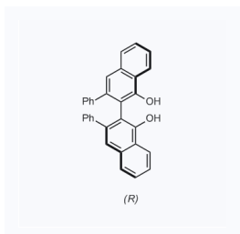
1156698 CAS: 147702-13-4
