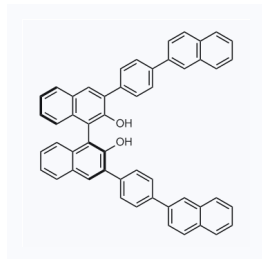
1157610 CAS: 309934-87-0
