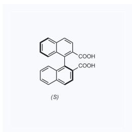
1161440 CAS: 18531-96-9
