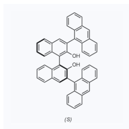
1156700 现货 CAS: 361342-50-9
