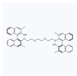
1163973 CAS: 1260243-73-9
