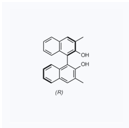
1157612 CAS: 55515-98-5
