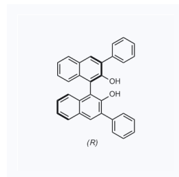
1157008 CAS: 75684-93-4
