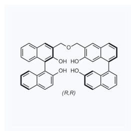
1157847 CAS: 265116-85-6
