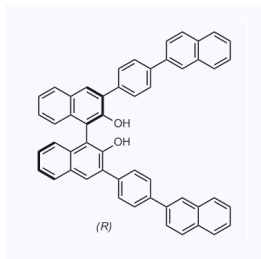
1157609 CAS: 309934-86-9
