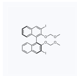
1157097 现货 CAS: 219583-87-6
