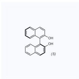
1024345 CAS: 18531-99-2
