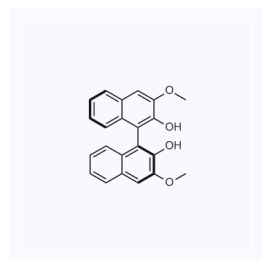
1167260 CAS: 151377-90-1
