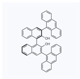
1157004 现货 CAS: 361342-49-6
