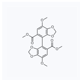
1066541 CAS: 73536-69-3
