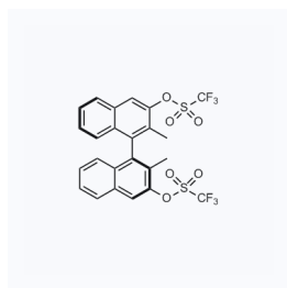
1167263 CAS: 326793-21-9
