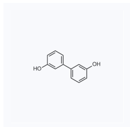
1159206 CAS: 612-76-0
