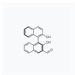
1158217 CAS: 345659-34-9
