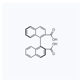
1134048 CAS: 99827-46-0
