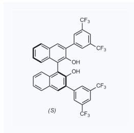
1157185 现货 CAS: 849939-13-5
