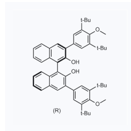
1158591 CAS: 1353682-93-5
