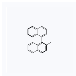
1158967 CAS: 118018-45-4
