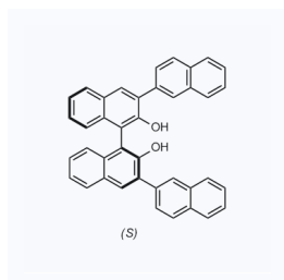
1157446 现货 CAS: 863659-89-6
