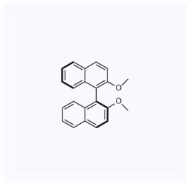
1156344 CAS: 75640-87-8
