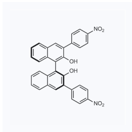
1111000 CAS: 945852-58-4
