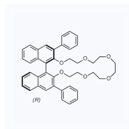
1162133 CAS: 75684-74-1
