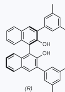
1157596 CAS: 215433-51-5
