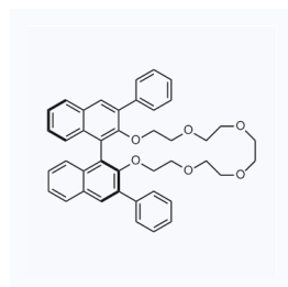
1162138 CAS: 75684-75-2
