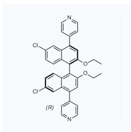
1158971 CAS: 431043-34-4
