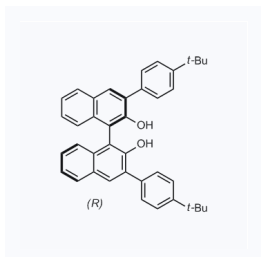
1157686 现货 CAS: 851615-06-0
