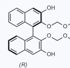
1167259 CAS: 1523248-61-4
