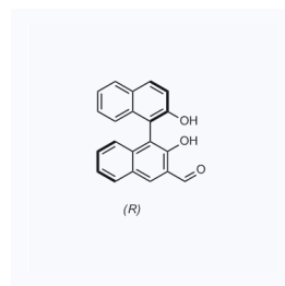
1158221 CAS: 349149-08-2
