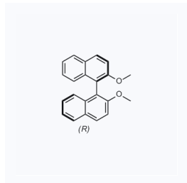
1155819 CAS: 35294-28-1
