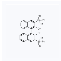
1156696 现货 CAS: 111822-69-6
