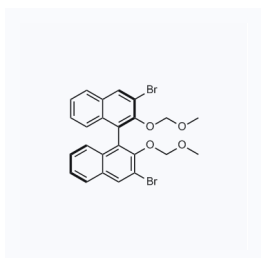
1157284 现货 CAS: 211734-49-5
