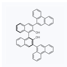
1157014 CAS: 957111-25-0
