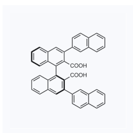
1167245 CAS: 1791455-29-2
