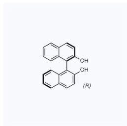
1024343 CAS: 18531-94-7
