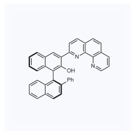
1166238 CAS: 1621903-81-8
