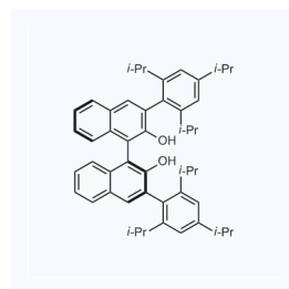
1067041 现货 CAS: 908338-44-3
