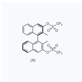
1167264 CAS: 625124-43-8
