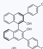
1158603 CAS: 851615-05-9
