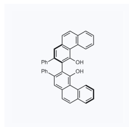
1155817 现货 CAS: 147702-15-6
