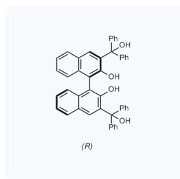
1157434 CAS: 336185-31-0
