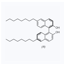
1167250 CAS: 208942-84-1
