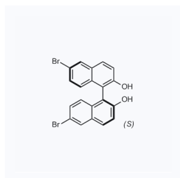
1044047 现货 CAS: 80655-81-8
