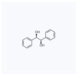
1034534 CAS: 52340-78-0
