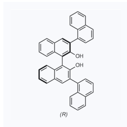
1157442 CAS: 851615-07-1
