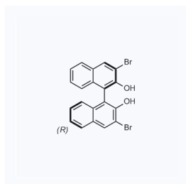
1016961 现货 CAS: 111795-43-8
