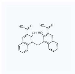
1019490 CAS: 130-85-8
