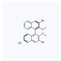
1042155 现货 CAS: 75714-59-9
