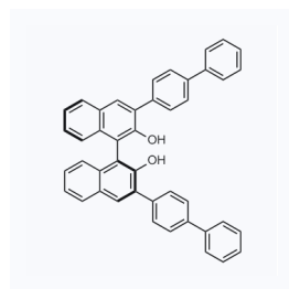
1157599 CAS: 220486-43-1
