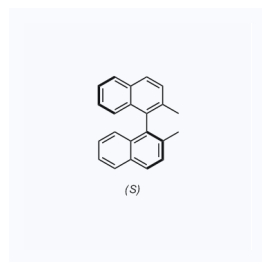
1156518 CAS: 32587-64-7
