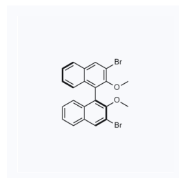
1042156 现货 CAS: 75714-60-2
