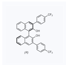
1157860 现货 CAS: 791616-58-5
