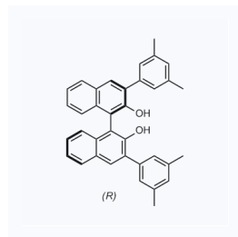
1157596 CAS: 215433-51-5
