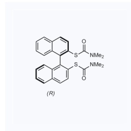
1167474 CAS: 147923-23-7
