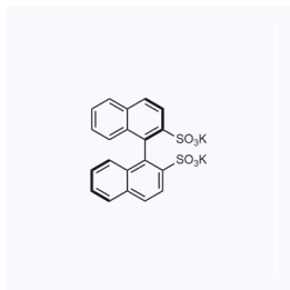
1178143 CAS: 1092934-19-4
