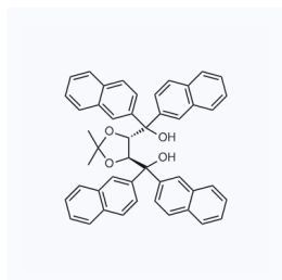
1163814 CAS: 137365-16-3
