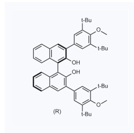
1158591 CAS: 1353682-93-5
