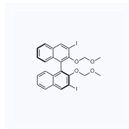
1157097 现货 CAS: 219583-87-6
