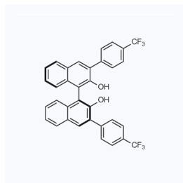
1161779 现货 CAS: 1621066-21-4
