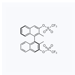
1167263 CAS: 326793-21-9
