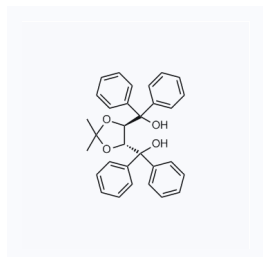
1046963 现货 CAS: 93379-48-7
