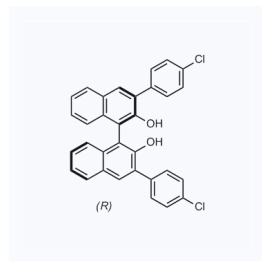
1158603 CAS: 851615-05-9
