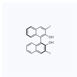
1157855 现货 CAS: 615247-86-4
