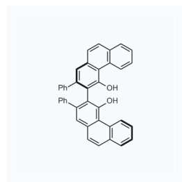
1155817 现货 CAS: 147702-15-6
