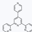
1156447 CAS: 112881-51-3
