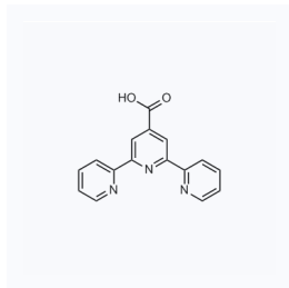
1021903 现货 CAS: 148332-36-9
