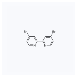
1024331 现货 CAS: 18511-71-2
