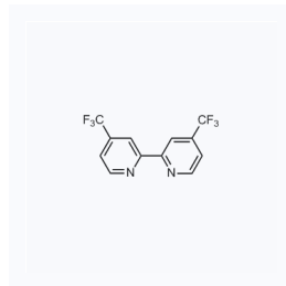
1152169 现货 CAS: 142946-79-0
