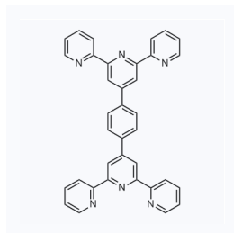
1021723 现货 CAS: 146406-75-9
