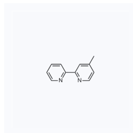
1092553 现货 CAS: 56100-19-7
