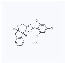
1158949 现货 CAS: 1214711-48-4
