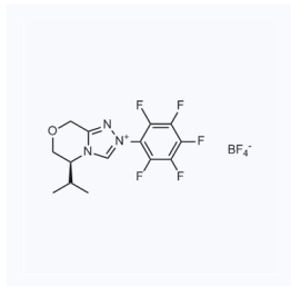
1158563 现货 CAS: 1431323-18-0
