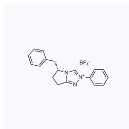
1161816 CAS: 463326-92-3
