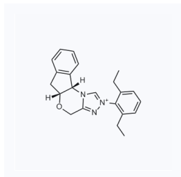
1174044 现货 CAS: 1221487-75-7
