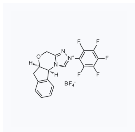
1157067 现货 CAS: 872143-57-2
