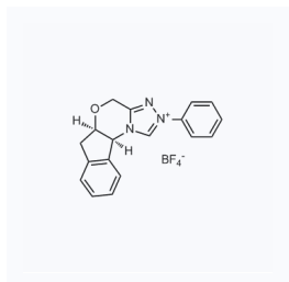
1157798 现货 CAS: 925706-36-1
