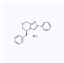
1060243 现货 CAS: 464174-87-6
