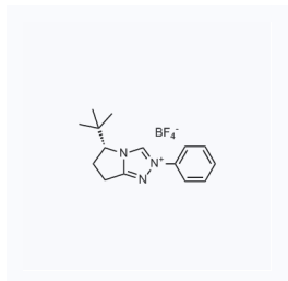
1163861 现货 CAS: 1448816-61-2
