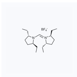
1176863 CAS: 1204324-18-4
