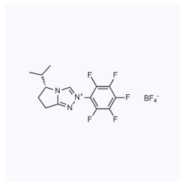
1163552 CAS: 1175052-07-9
