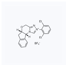
1158584 现货 CAS: 1787246-78-9
