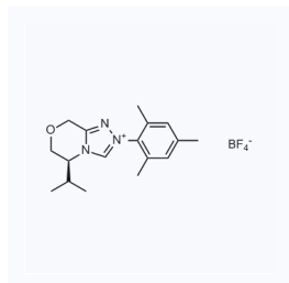
1158581 现货 CAS: 1631733-83-9
