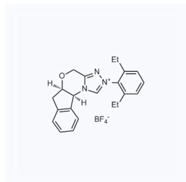
1158953 现货 CAS: 1221487-76-8
