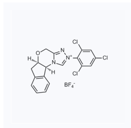
1158951 现货 CAS: 1252006-72-6
