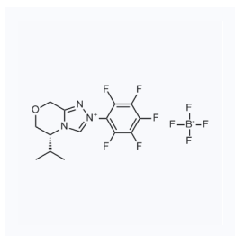
1186102 CAS: 2254501-59-0
