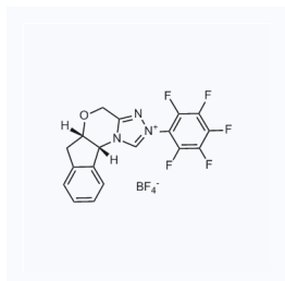
1156993 现货 CAS: 740816-14-2
