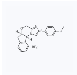
1158965 现货 CAS: 941283-79-0
