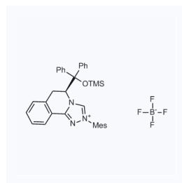
1164274 CAS: 1710476-21-3
