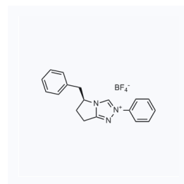
1174092 CAS: 960254-94-8
