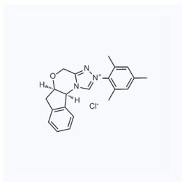
1155794 CAS: 903571-02-8
