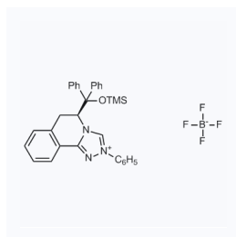
1174041 CAS: 1710476-13-3
