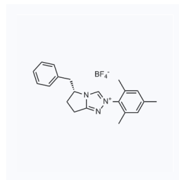
1163867 CAS: 1469801-67-9
