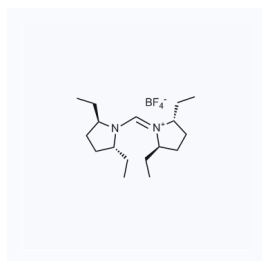
1176864 CAS: 1204324-20-8
