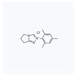
1173937 CAS: 862893-81-0
