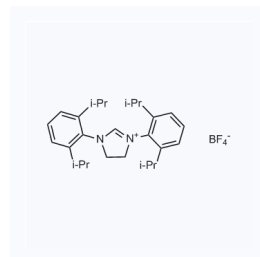
1105802 现货 CAS: 282109-83-5
