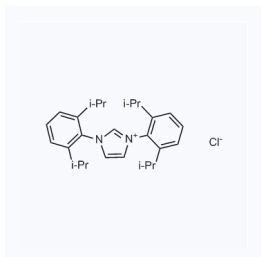
1027265 现货 CAS: 250285-32-6
