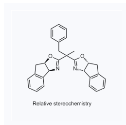
1215717 CAS: 2101474-75-1
