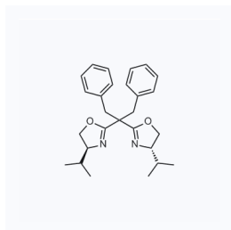
1158182 CAS: 444575-98-8
