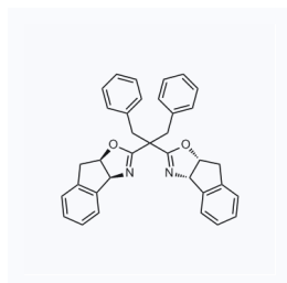
1134691 CAS: 195703-68-5
