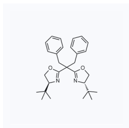
1168525 CAS: 319489-90-2
