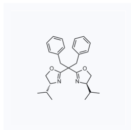
1158185 CAS: 880479-99-2
