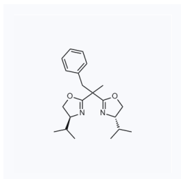
1215738 CAS: 698350-53-7
