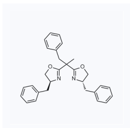
1215720 CAS: 1615699-79-0
