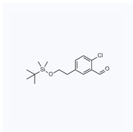
1173648 现货 CAS: 1911653-47-8
