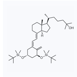
1057296 现货 CAS: 140710-96-9
