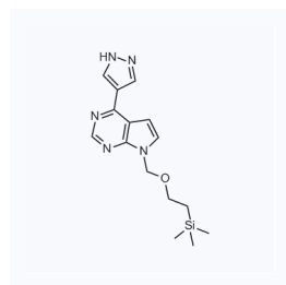
1049345 现货 CAS: 941685-27-4
