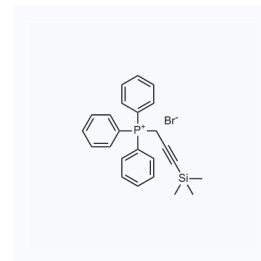
1190608 CAS: 42134-49-6
