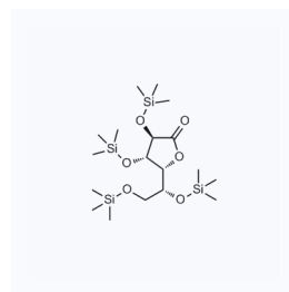
1169959 CAS: 2348-31-4
