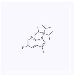
1075304 CAS: 928653-76-3
