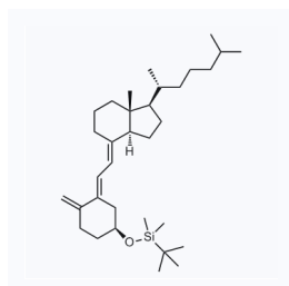
1058182 现货 CAS: 87649-55-6
