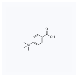
1115954 现货 CAS: 15290-29-6
