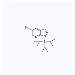
1048881 现货 CAS: 858116-66-2
