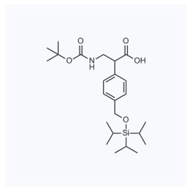
1159223 CAS: 1253955-24-6
