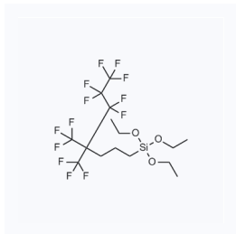
1192349 CAS: 130676-81-2
