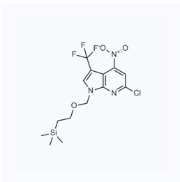
1059783 CAS: 892414-51-6
