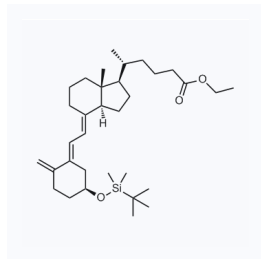
1077923 CAS: 147125-14-2
