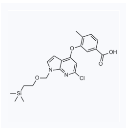
1057507 CAS: 1415564-64-5
