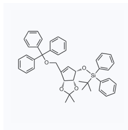
1061191 现货 CAS: 2241016-47-5
