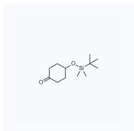
1183744 现货 CAS: 55145-45-4
