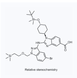
1057757 CAS: 1415565-14-8
