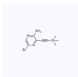
1061109 现货 CAS: 875781-41-2
