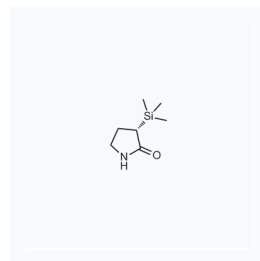
1057177 CAS: 406497-08-3
