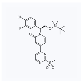
1084446 CAS: 1453851-69-8
