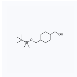
1049240 现货 CAS: 141836-50-2
