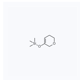
1128935 CAS: 82272-08-0
