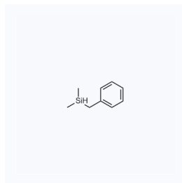
1200231 CAS: 1631-70-5
