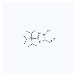
1165278 CAS: 1134560-73-8
