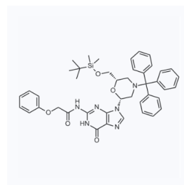
1173554 CAS: 1370348-31-4
