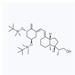
1163224 CAS: 139239-33-1
