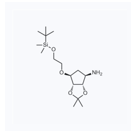
1059493 现货 CAS: 1400665-85-1
