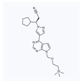
1078250 CAS: 941685-40-1
