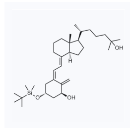
1057535 CAS: 132054-64-9
