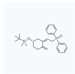
1058427 现货 CAS: 100858-27-3
