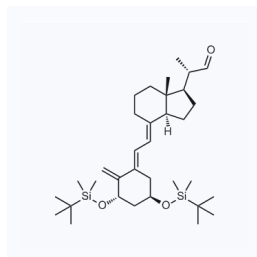
1058838 现货 CAS: 112828-13-4
