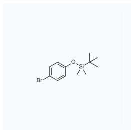
1039737 现货 CAS: 67963-68-2
