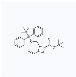
1119077 CAS: 1638771-11-5
