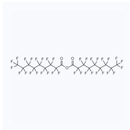
1192233 CAS: 228407-54-3
