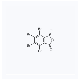
1038578 CAS: 632-79-1
