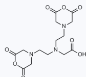
1026849 CAS: 23911-26-4
