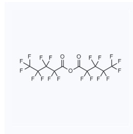
1192118 CAS: 308-28-1
