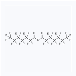
1192202 CAS: 78225-99-7
