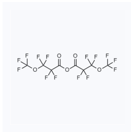
1192330 CAS: 42566-65-4
