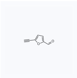
1192989 CAS: 153026-71-2
