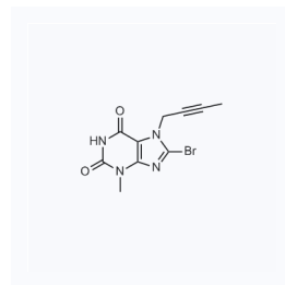
1060373 现货 CAS: 666816-98-4
