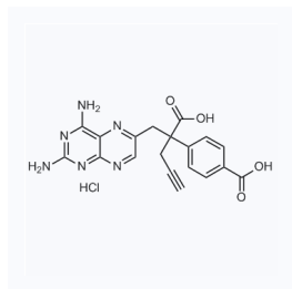
1061918 现货 CAS: 1497287-42-9
