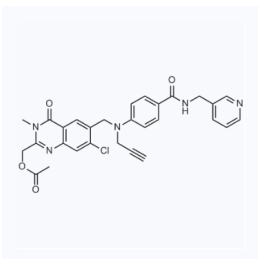
1057584 现货 CAS: 1258400-23-5
