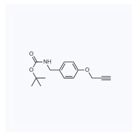
1060202 现货 CAS: 1380401-33-1
