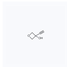
1122015 CAS: 1352492-38-6
