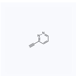
1122013 CAS: 1017793-08-6
