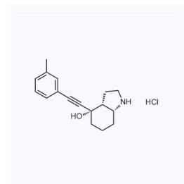
1061288 现货 CAS: 1636881-76-9
