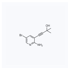
1066864 现货 CAS: 1262985-25-0
