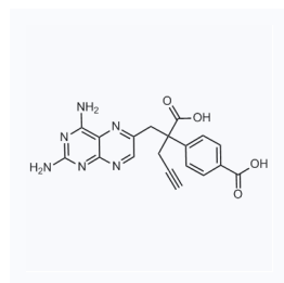
1058178 现货 CAS: 146464-92-8
