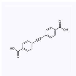
1053060 现货 CAS: 16819-43-5
