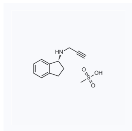
1022901 现货 CAS: 161735-79-1
