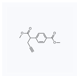
1058169 现货 CAS: 146464-90-6
