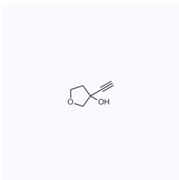
1122014 CAS: 137344-86-6
