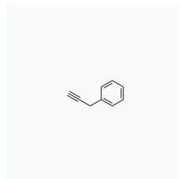
1183211 CAS: 10147-11-2
