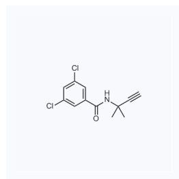
1084007 现货 CAS: 23950-58-5
