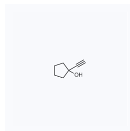
1023707 CAS: 17356-19-3
