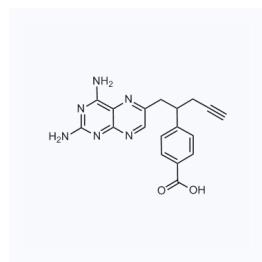
1057367 现货 CAS: 146464-93-9
