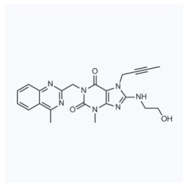
1060381 现货 CAS: 2074688-84-7
