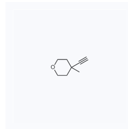
1121509 CAS: 1363382-15-3
