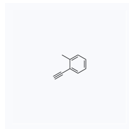
1042539 CAS: 766-47-2
