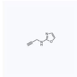
1165479 CAS: 1899056-77-9
