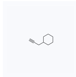
1023942 CAS: 17715-00-3
