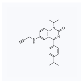
1058330 现货 CAS: 478963-46-1
