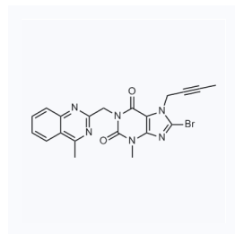
1060375 现货 CAS: 853029-57-9
