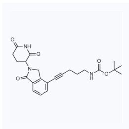
1181260 现货 CAS: 2136248-15-0
