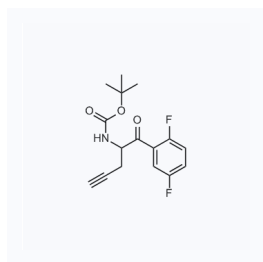
1047965 现货 CAS: 1172623-96-9
