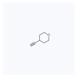
1121507 CAS: 1202245-65-5
