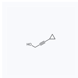
1122025 CAS: 101974-69-0
