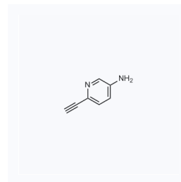
1145949 CAS: 1256824-94-8
