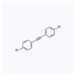
1062350 现货 CAS: 2789-89-1
