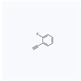
1042541 CAS: 766-49-4
