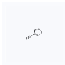
1039525 CAS: 67237-53-0
