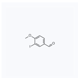
1111979 现货 CAS: 2314-37-6
