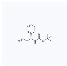
1069362 现货 CAS: 135865-78-0
