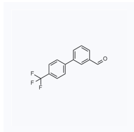
1068695 现货 CAS: 343604-24-0
