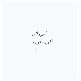
1065280 现货 CAS: 153034-82-3
