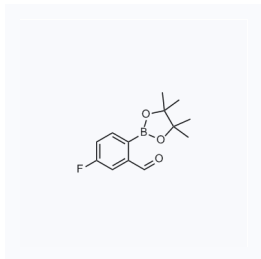
1166704 现货 CAS: 943310-52-9
