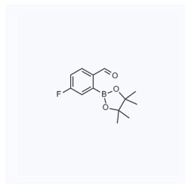
1112083 现货 CAS: 1844839-22-0
