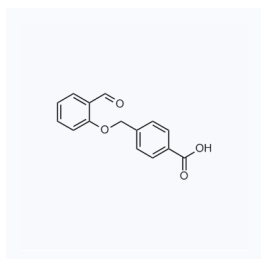
1057016 现货 CAS: 338994-68-6
