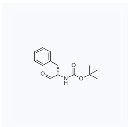
1040795 现货 CAS: 72155-45-4
