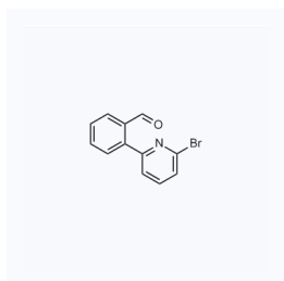
1167151 现货 CAS: 914349-51-2
