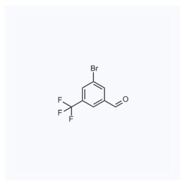
1033344 现货 CAS: 477535-41-4
