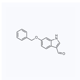
1069181 现货 CAS: 92855-64-6
