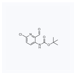
1118696 现货 CAS: 1199557-04-4
