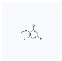
1138531 现货 CAS: 111829-72-2
