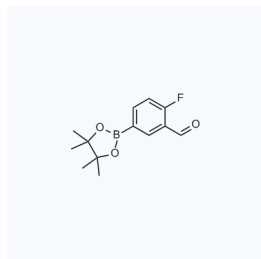
1167685 现货 CAS: 443776-94-1
