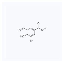
1173283 现货 CAS: 706820-79-3
