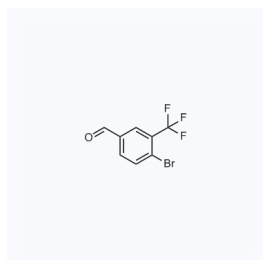
1068776 现货 CAS: 34328-47-7
