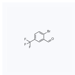
1015226 现货 CAS: 102684-91-3
