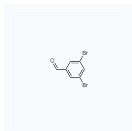
1036234 现货 CAS: 56990-02-4
