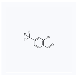
1062516 现货 CAS: 85118-24-7
