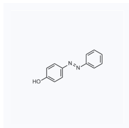
1023383 现货 CAS: 1689-82-3
