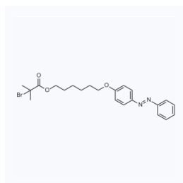
1181695 CAS: 951322-07-9
