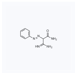
1066740 现货 CAS: 100607-08-7
