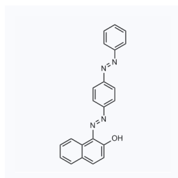
1044973 CAS: 85-86-9
