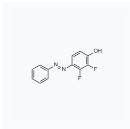
1044685 CAS: 847872-04-2
