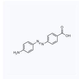
1207986 CAS: 6925-48-0
