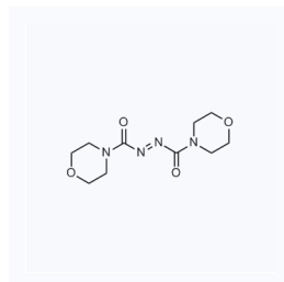
1015606 现货 CAS: 10465-82-4
