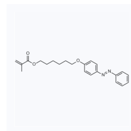
1181602 CAS: 169237-94-9
