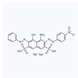
1015896 CAS: 1064-48-8
