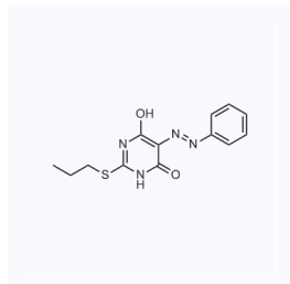
1061890 现货 CAS: 946855-76-1
