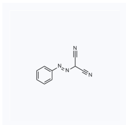
1059796 现货 CAS: 6017-21-6
