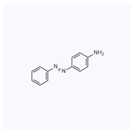
1147436 现货 CAS: 25548-34-9
