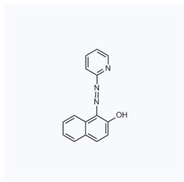
1044969 现货 CAS: 85-85-8
