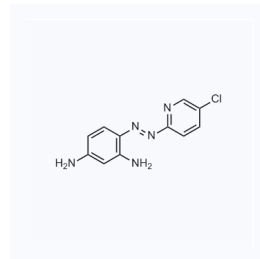
1029773 CAS: 33006-91-6
