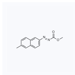
1179264 现货 CAS: 2138504-49-9
