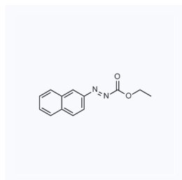
1179260 现货 CAS: 2138504-42-2
