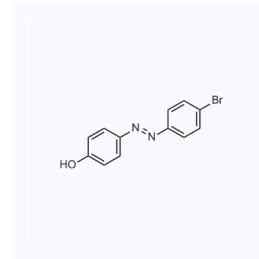
1028853 CAS: 3035-94-7
