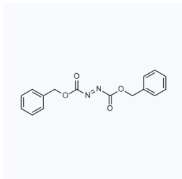
1027078 现货 CAS: 2449-05-0
