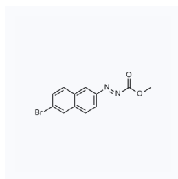
1179263 CAS: 2138504-50-2
