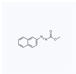
1179258 现货 CAS: 2138504-41-1
