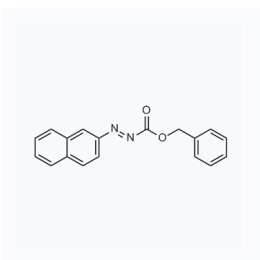
1179262 CAS: 2138504-44-4
