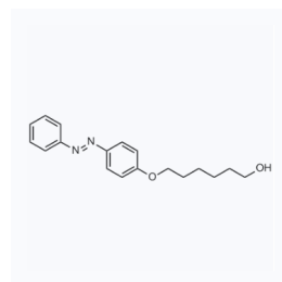
1181240 CAS: 162844-58-8
