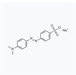
1148320 CAS: 547-58-0
