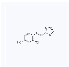
1026371 现货 CAS: 2246-46-0
