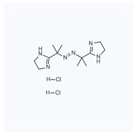
1065412 现货 CAS: 27776-21-2
