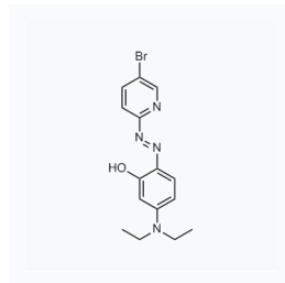
1199394 现货 CAS: 14337-53-2
