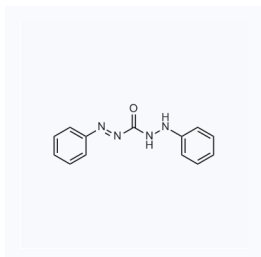
1203103 现货 CAS: 538-62-5
