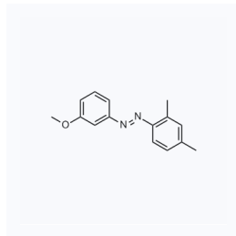
1051503 CAS: 1882034-29-8
