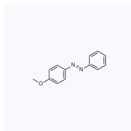
1026864 现货 CAS: 2396-60-3
