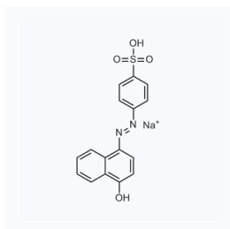
1086720 CAS: 523-44-4
