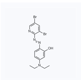
1021399 CAS: 14337-54-3
