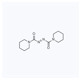
1015605 现货 CAS: 10465-81-3
