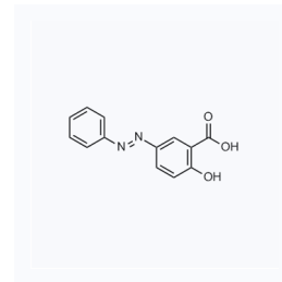
1029275 CAS: 3147-53-3
