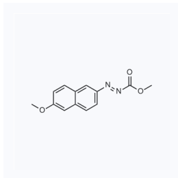
1179265 CAS: 2138504-48-8
