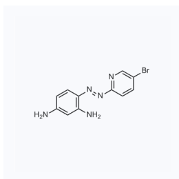
1034054 CAS: 50768-75-7
