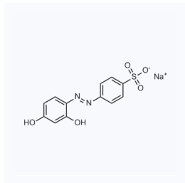
1080225 现货 CAS: 547-57-9
