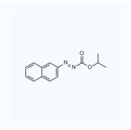
1179261 CAS: 2138504-43-3
