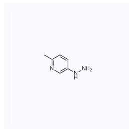
1088740 CAS: 197516-48-6
