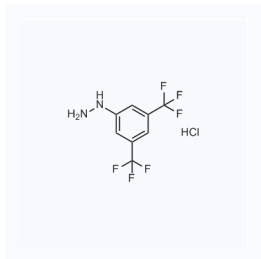
1033842 现货 CAS: 502496-23-3
