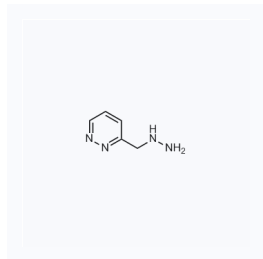
1127875 CAS: 1333245-18-3
