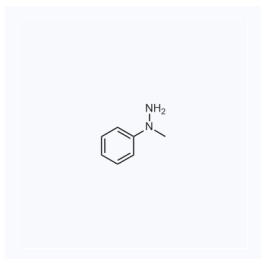
1074004 CAS: 618-40-6
