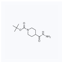
1053158 现货 CAS: 187834-88-4
