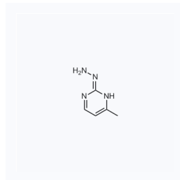
1116526 CAS: 63170-77-4
