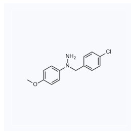
1059339 现货 CAS: 62646-04-2
