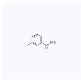
1035033 CAS: 536-89-0
