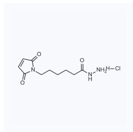
1069158 现货 CAS: 175290-73-0
