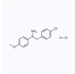
1076859 现货 CAS: 20955-94-6
