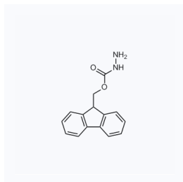
1065526 现货 CAS: 35661-51-9
