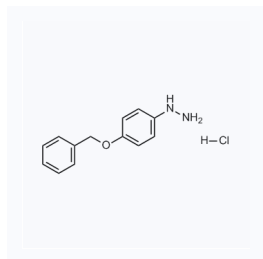
1066327 现货 CAS: 52068-30-1
