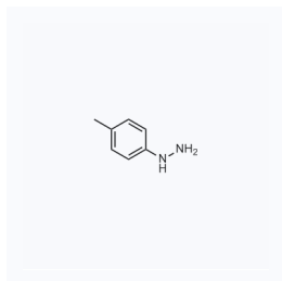
1181298 CAS: 539-44-6
