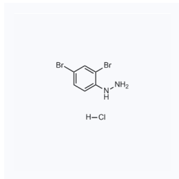
1130972 现货 CAS: 149998-17-4
