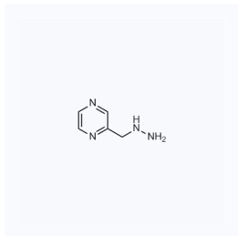
1124437 CAS: 887592-66-7
