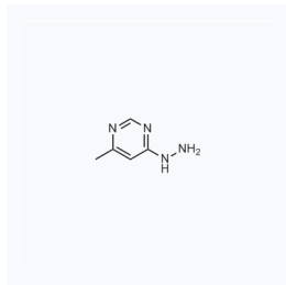
1116613 CAS: 33592-43-7
