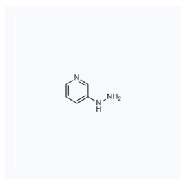
1093004 CAS: 42166-50-7
