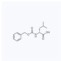
1066923 现货 CAS: 28862-79-5
