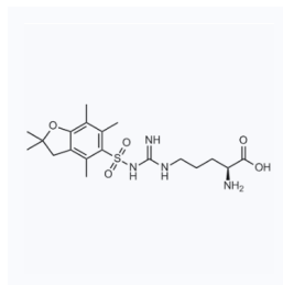
1069522 现货 CAS: 200115-86-2
