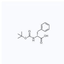
1024550 现货 CAS: 18942-49-9
