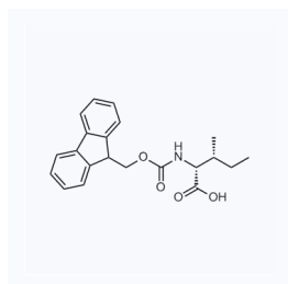
1021438 现货 CAS: 143688-83-9
