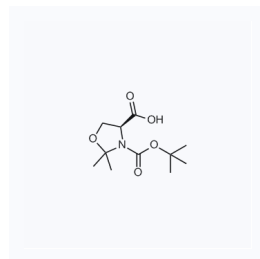
1173432 现货 CAS: 139009-66-8
