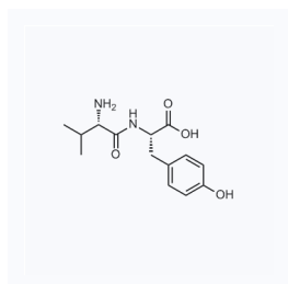
1028931 现货 CAS: 3061-91-4
