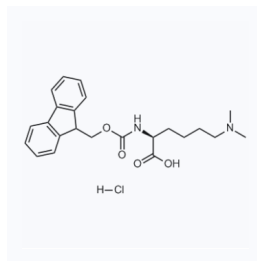
1075689 现货 CAS: 252049-10-8
