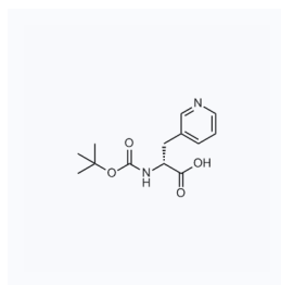
1047639 现货 CAS: 98266-33-2
