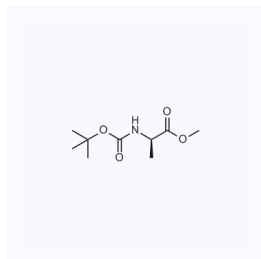
1046593 现货 CAS: 91103-47-8
