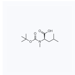
1045821 现货 CAS: 89536-84-5
