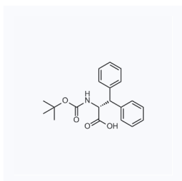
1021347 现货 CAS: 143060-31-5
