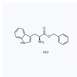
1064193 现货 CAS: 35858-81-2
