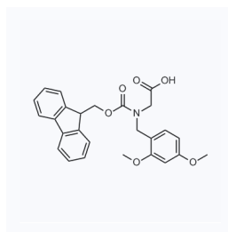
1170440 现货 CAS: 166881-42-1
