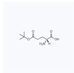
1032896 现货 CAS: 45125-00-6
