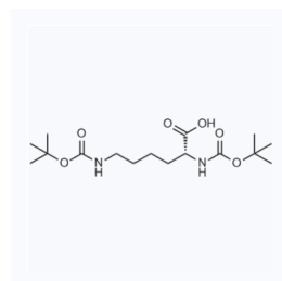
1066444 现货 CAS: 65360-27-2
