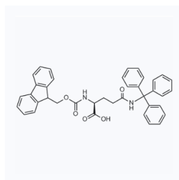
1019930 现货 CAS: 132327-80-1
