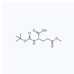
1062664 现货 CAS: 45214-91-3
