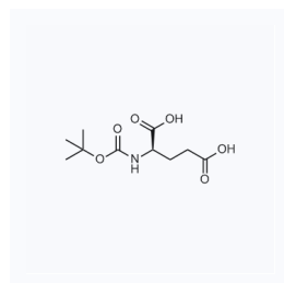
1167934 现货 CAS: 34404-28-9
