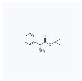
1069537 现货 CAS: 65715-93-7
