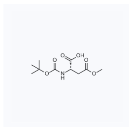
1037097 现货 CAS: 59768-74-0
