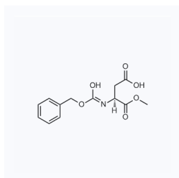
1033147 现货 CAS: 4668-42-2
