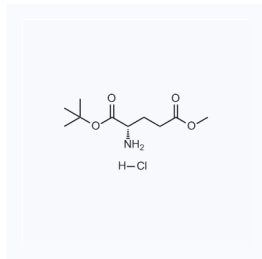
1137754 现货 CAS: 34582-33-7
