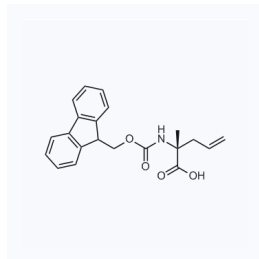
1063582 现货 CAS: 288617-76-5
