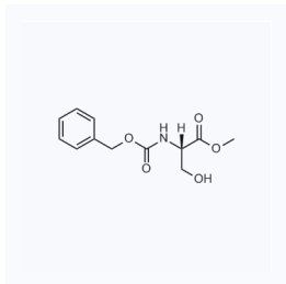
1023298 现货 CAS: 1676-81-9
