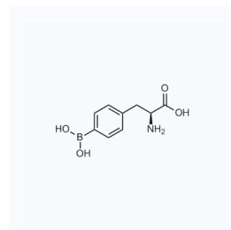
1199258 现货 CAS: 76410-58-7
