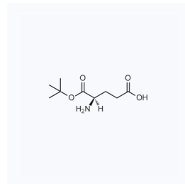
1063557 现货 CAS: 25456-76-2
