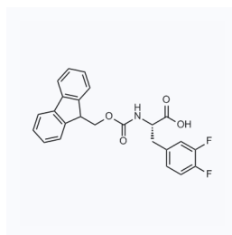
1025016 现货 CAS: 198560-43-9
