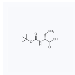
1041024 现货 CAS: 73259-81-1
