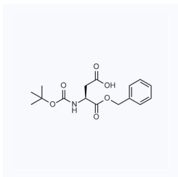
1029134 现货 CAS: 30925-18-9
