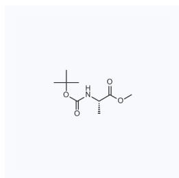
1028425 现货 CAS: 28875-17-4
