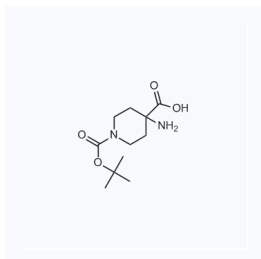
1024254 现货 CAS: 183673-71-4
