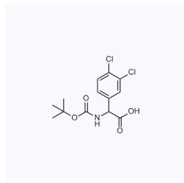
1165025 现货 CAS: 142121-95-7
