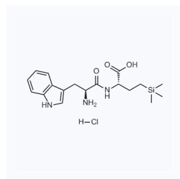
1093259 现货 CAS: 1093259
