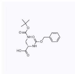
1023433 现货 CAS: 16947-84-5
