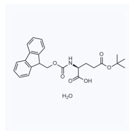
1025308 现货 CAS: 204251-24-1
