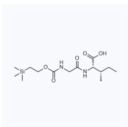
1164556 现货 CAS: 863658-70-2
