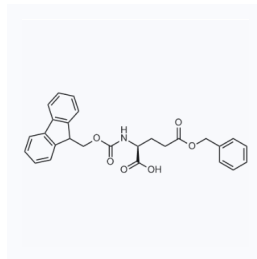
1018711 现货 CAS: 123639-61-2
