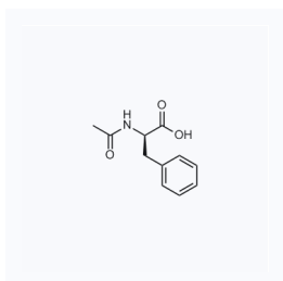
1015062 现货 CAS: 10172-89-1
