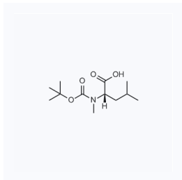
1034927 现货 CAS: 53363-89-6
