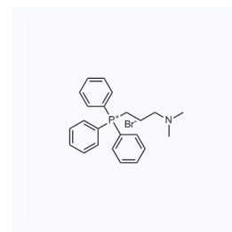
1024246 CAS: 18355-96-9
