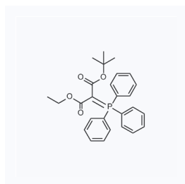
1057239 CAS: 157188-20-0
