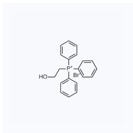
1165096 CAS: 7237-34-5
