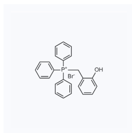
1203206 CAS: 70340-04-4
