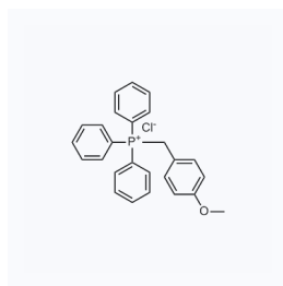
1030310 CAS: 3462-97-3
