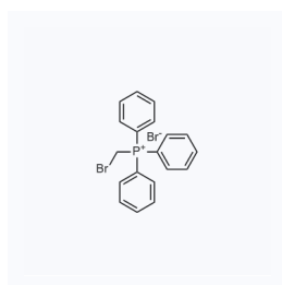
1015388 CAS: 1034-49-7
