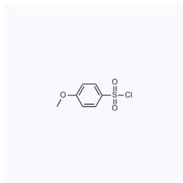
1047683 现货 CAS: 98-68-0
