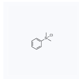
1042621 现货 CAS: 768-33-2
