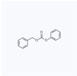
1047908 CAS: 28170-07-2
