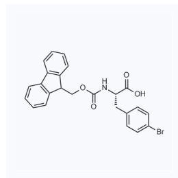
1025018 现货 CAS: 198561-04-5
