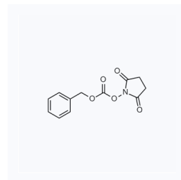
1019685 现货 CAS: 13139-17-8
