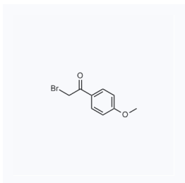
1027789 现货 CAS: 2632-13-5
