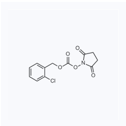
1039274 CAS: 65853-65-8
