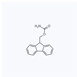
1044598 现货 CAS: 84418-43-9
