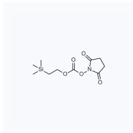
1062662 现货 CAS: 78269-85-9
