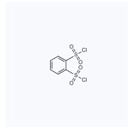
1039015 CAS: 6461-76-3
