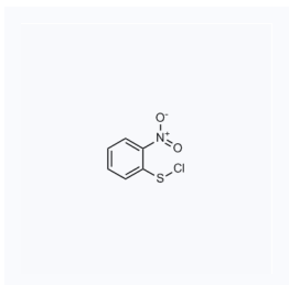
1057370 现货 CAS: 7669-54-7
