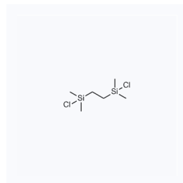
1085912 现货 CAS: 13528-93-3
