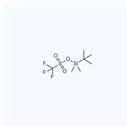
1040228 现货 CAS: 69739-34-0
