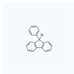
1035614 现货 CAS: 55135-66-5
