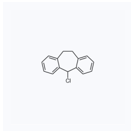
1115990 CAS: 1210-33-9
