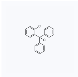
1032431 CAS: 42074-68-0
