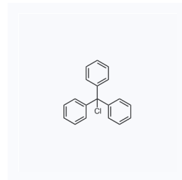
1042622 现货 CAS: 76-83-5
