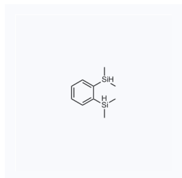
1024081 现货 CAS: 17985-72-7
