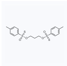
1031536 CAS: 3866-79-3
