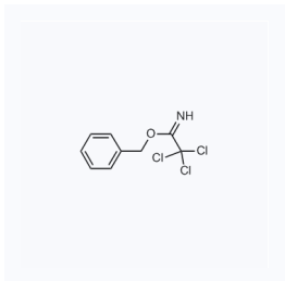
1044209 现货 CAS: 81927-55-1
