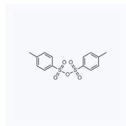
1062140 现货 CAS: 4124-41-8
