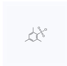
1042835 现货 CAS: 773-64-8
