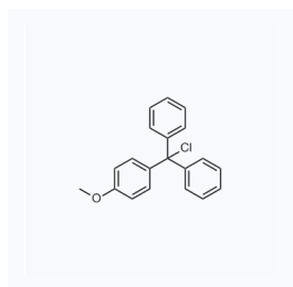
1021552 现货 CAS: 14470-28-1
