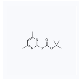
1149350 CAS: 41840-28-2
