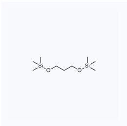
1024040 CAS: 17887-80-8
