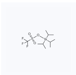
1061071 现货 CAS: 80522-42-5
