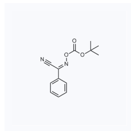
1036726 现货 CAS: 58632-95-4
