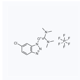
1029798 现货 CAS: 330645-87-9
