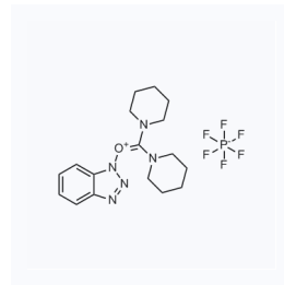
1025497 CAS: 206752-41-2
