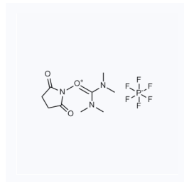
1027850 现货 CAS: 265651-18-1
