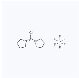
1205865 现货 CAS: 135540-11-3
