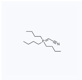
1116740 现货 CAS: 157141-27-0
