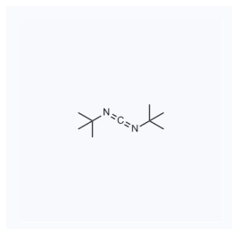
1193228 现货 CAS: 691-24-7
