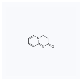
1035355 现货 CAS: 5439-14-5
