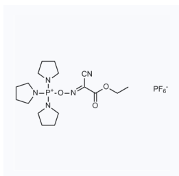
1138675 现货 CAS: 153433-21-7
