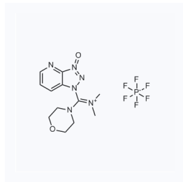
1205872 CAS: 958029-37-3
