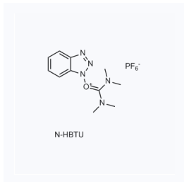
1047164 现货 CAS: 94790-37-1
