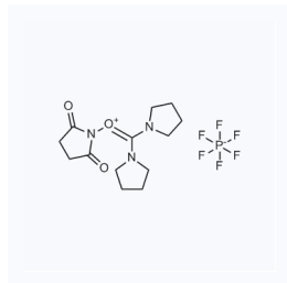
1025562 现货 CAS: 207683-26-9
