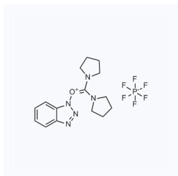
1015705 现货 CAS: 105379-24-6
