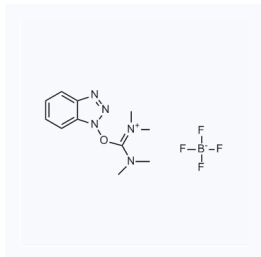
1018989 现货 CAS: 125700-67-6
