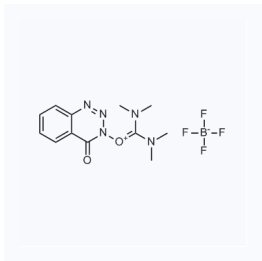
1018990 CAS: 125700-69-8
