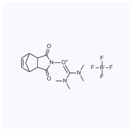
1018992 现货 CAS: 125700-73-4
