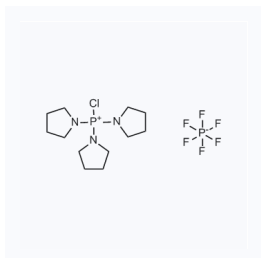
1205868 现货 CAS: 133894-48-1
