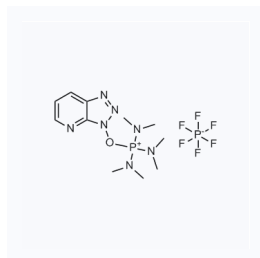
1022565 现货 CAS: 156311-85-2
