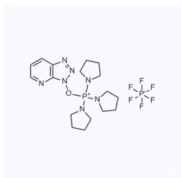
1022563 现货 CAS: 156311-83-0
