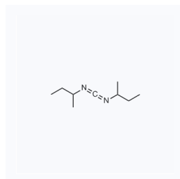
1193227 现货 CAS: 66006-67-5
