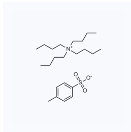
1040729 CAS: 7182-86-7
