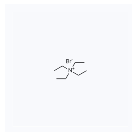
1040739 CAS: 71-91-0
