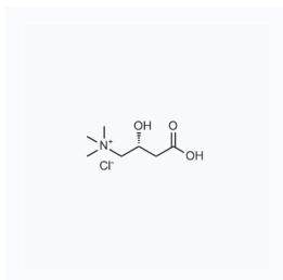
1039414 现货 CAS: 6645-46-1
