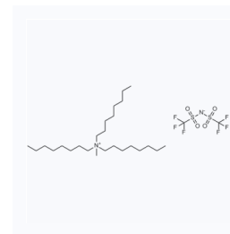
1031192 CAS: 375395-33-8
