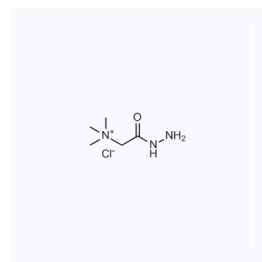
1180236 CAS: 123-46-6
