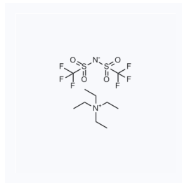
1200196 CAS: 161401-26-9
