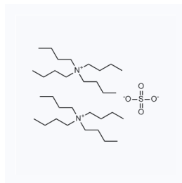
1183747 CAS: 2472-88-0
