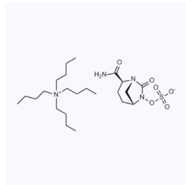
1061092 现货 CAS: 1192651-80-1
