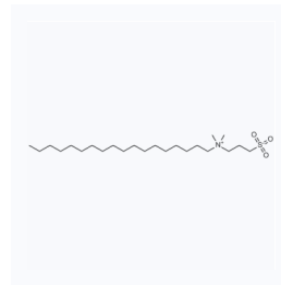
1019858 CAS: 13177-41-8
