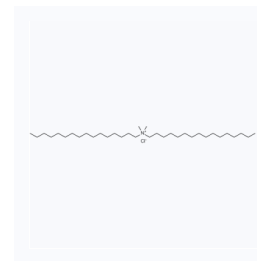
1137781 CAS: 1812-53-9
