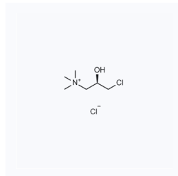
1173262 现货 CAS: 117604-42-9
