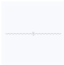
1016149 CAS: 107-64-2
