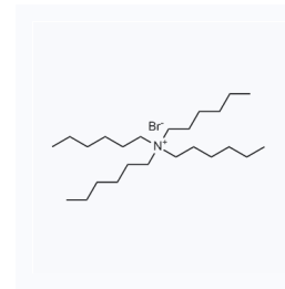
1032642 CAS: 4328-13-6
