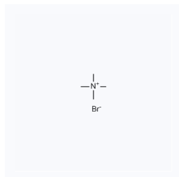
1038923 现货 CAS: 64-20-0
