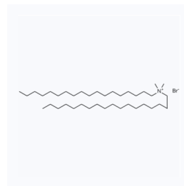
1199429 CAS: 3700-67-2
