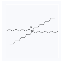
1021936 现货 CAS: 14866-33-2
