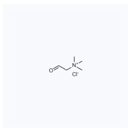
1042928 CAS: 7758-31-8
