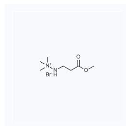
1147059 CAS: 106966-25-0
