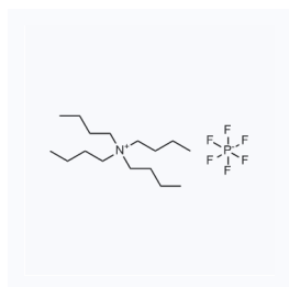
1029168 现货 CAS: 3109-63-5
