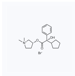
1191426 CAS: 129784-11-8
