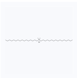
1040494 CAS: 70755-47-4
