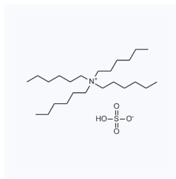
1208213 CAS: 32503-34-7
