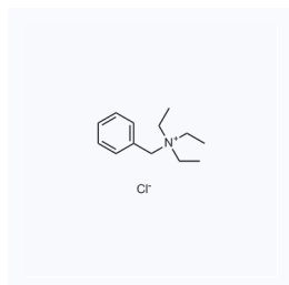
1036027 现货 CAS: 56-37-1
