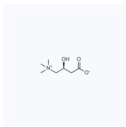
1035224 CAS: 541-14-0
