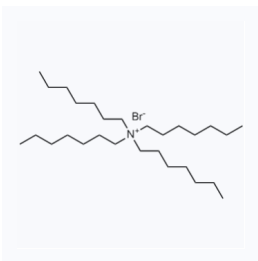
1032689 CAS: 4368-51-8
