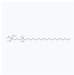
1028143 CAS: 27668-52-6
