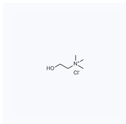
1083195 现货 CAS: 67-48-1
