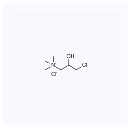
1029880 现货 CAS: 3327-22-8
