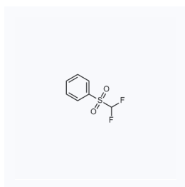
1022369 现货 CAS: 1535-65-5
