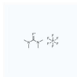
1023070 现货 CAS: 164298-23-1
