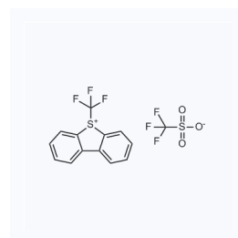
1019320 现货 CAS: 129946-88-9
