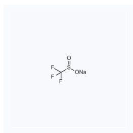
1062030 现货 CAS: 2926-29-6
