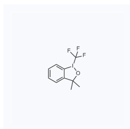
1062115 现货 CAS: 887144-97-0
