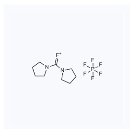
1023071 现货 CAS: 164298-25-3
