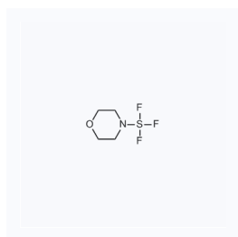
1034130 现货 CAS: 51010-74-3
