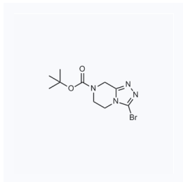
1047979 现货 CAS: 723286-80-4
