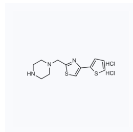
1146453 CAS: 1177319-77-5
