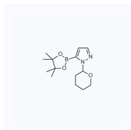
1046445 现货 CAS: 903550-26-5
