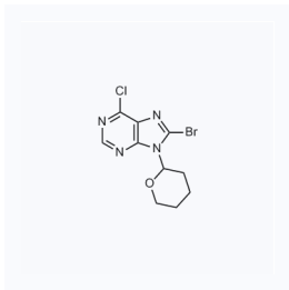
1120598 CAS: 218431-08-4
