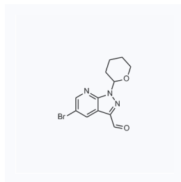
1177176 CAS: 1314734-59-2
