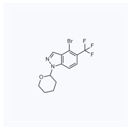
1166392 CAS: 2044704-81-4
