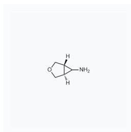
1126228 现货 CAS: 1048962-48-6
