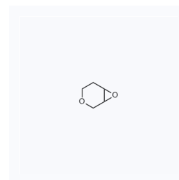
1122229 现货 CAS: 286-22-6
