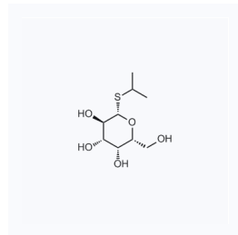
1079582 现货 CAS: 367-93-1
