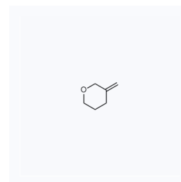
1140254 现货 CAS: 88073-01-2
