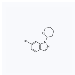
1126081 现货 CAS: 1158680-88-6
