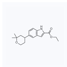
1114806 现货 CAS: 2212021-76-4
