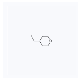
1051648 现货 CAS: 101691-94-5
