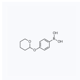
1024173 现货 CAS: 182281-01-2
