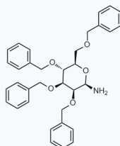
1163448 CAS: 150370-50-6
