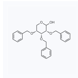
1135388 CAS: 20787-21-7
