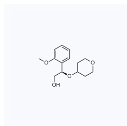
1090375 现货 CAS: 1434652-66-0
