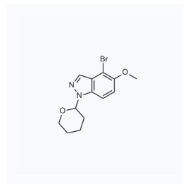
1166317 CAS: 2158298-59-8
