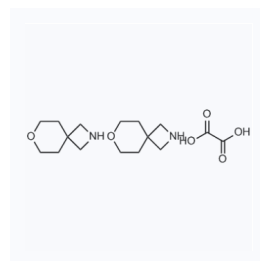
1120631 CAS: 1523571-04-1
