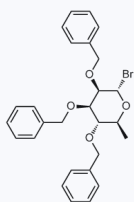
1163916 CAS: 59055-61-7
