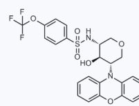
1176365 CAS: 2088956-23-2
