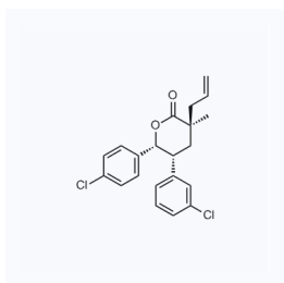
1081938 CAS: 1352076-45-9
