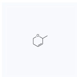
1140235 现货 CAS: 55230-25-6
