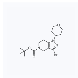
1175139 CAS: 1936429-15-0
