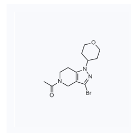
1159824 CAS: 1936429-16-1
