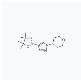
1050652 现货 CAS: 1040377-03-4
