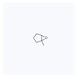
1182922 现货 CAS: 16240-42-9
