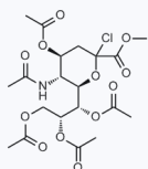
1060251 CAS: 132883-18-2
