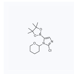
1122622 CAS: 1029684-36-3
