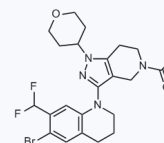
1176215 CAS: 1936429-30-9
