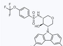
1176367 CAS: 2088956-21-0
