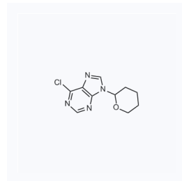
1040991 现货 CAS: 7306-68-5
