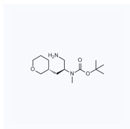
1048708 现货 CAS: 942145-27-9
