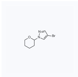
1124623 现货 CAS: 82099-98-7
