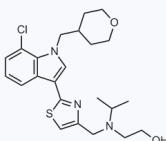
1098478 CAS: 865712-14-7
