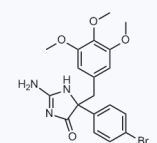
1192454 CAS: 1354918-47-0
