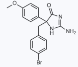
1192435 CAS: 1354936-25-6
