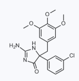
1192444 CAS: 1354925-02-2
