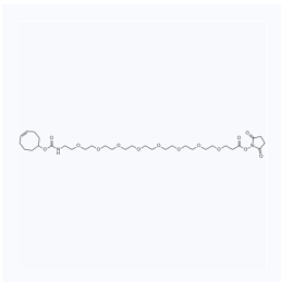
1185315 CAS: 2353409-95-5
