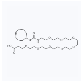
1185266 CAS: 2353410-03-2
