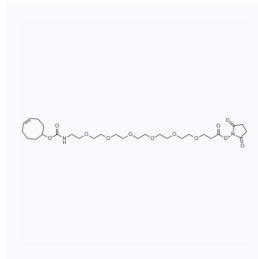
1185314 CAS: 2353409-96-6
