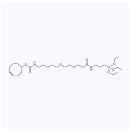
1185824 CAS: 2250217-32-2
