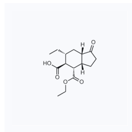
1057627 现货 CAS: 130274-13-4
