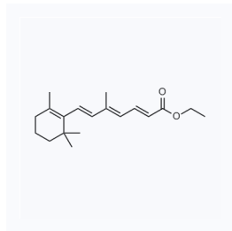
1067008 现货 CAS: 74109-37-8
