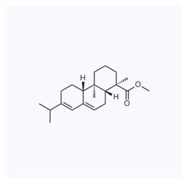
1019155 CAS: 127-25-3
