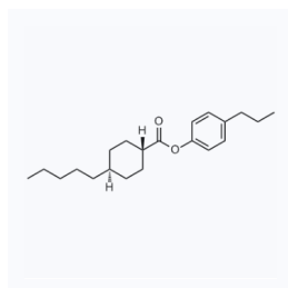
1039642 CAS: 67589-71-3
