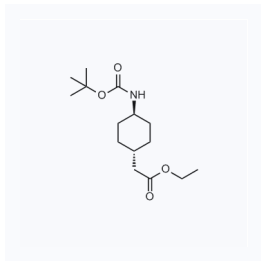
1078563 现货 CAS: 946598-34-1
