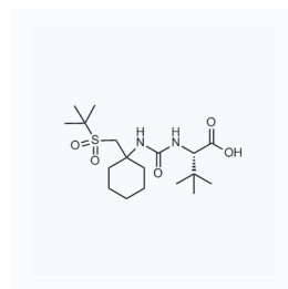
1057622 现货 CAS: 1208245-85-5
