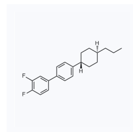
1044893 CAS: 85312-59-0
