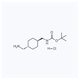
1201304 CAS: 256649-59-9
