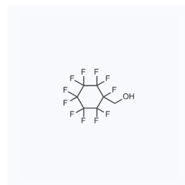
1192182 CAS: 28788-68-3
