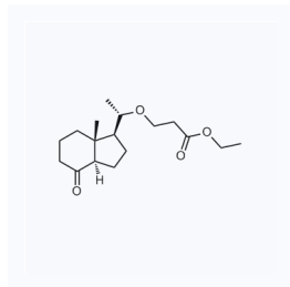
1058991 CAS: 413571-28-5
