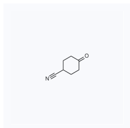
1061571 现货 CAS: 34916-10-4
