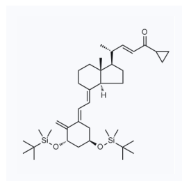
1056975 现货 CAS: 112849-17-9
