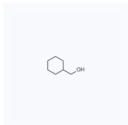
1014767 现货 CAS: 100-49-2
