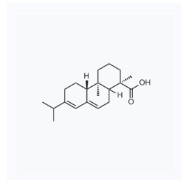
1034262 CAS: 514-10-3
