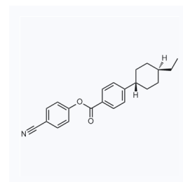
1045790 CAS: 89331-97-5
