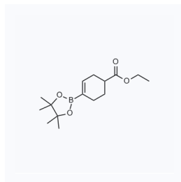
1064438 现货 CAS: 1049004-32-1
