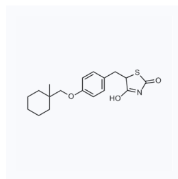
1041808 现货 CAS: 74772-77-3
