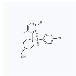
1057249 CAS: 656810-84-3
