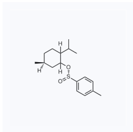
1046727 CAS: 91796-57-5
