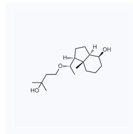
1067310 现货 CAS: 192573-37-8
