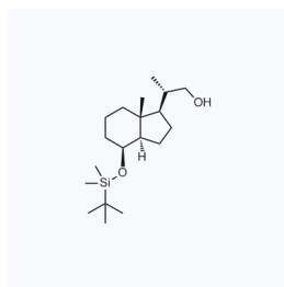
1075776 现货 CAS: 100928-03-8
