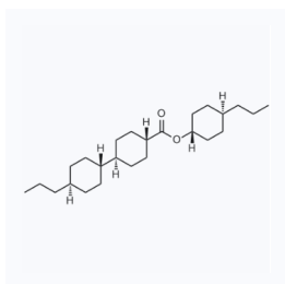
1044440 CAS: 83242-83-5
