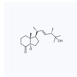
1058986 CAS: 95716-68-0
