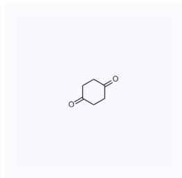
1038750 现货 CAS: 637-88-7
