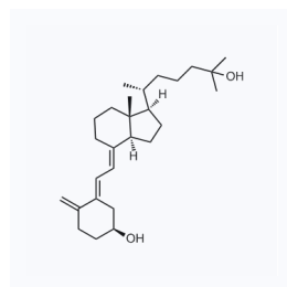
1058989 CAS: 1233749-00-2
