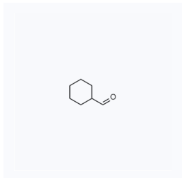
1092674 现货 CAS: 2043-61-0
