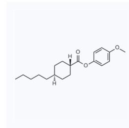
1039640 CAS: 67589-52-0
