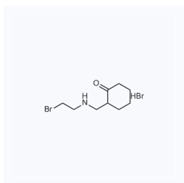
1142799 CAS: 479192-79-5
