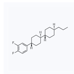
1044388 CAS: 82832-57-3
