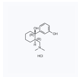
1021895 CAS: 148262-77-5
