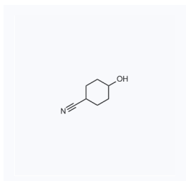
1053017 现货 CAS: 24056-34-6
