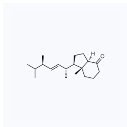
1076016 现货 CAS: 55812-80-1
