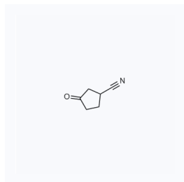
1106099 CAS: 41171-91-9
