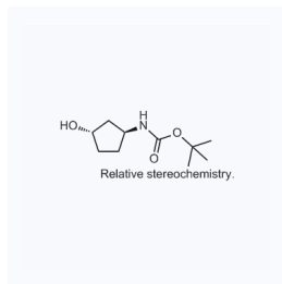
1129183 现货 CAS: 207729-04-2
