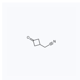
1122919 现货 CAS: 2007916-61-0
