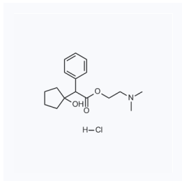
1036745 现货 CAS: 5870-29-1
