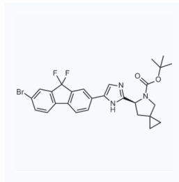
1060320 现货 CAS: 1441670-89-8
