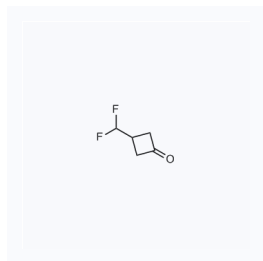
1122333 现货 CAS: 1461713-56-3
