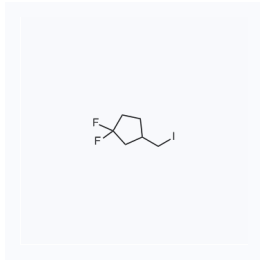
1128631 CAS: 1042153-28-5
