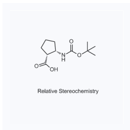
1124785 现货 CAS: 136315-70-3
