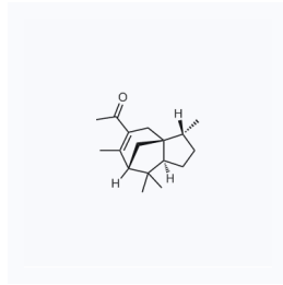
1029560 CAS: 32388-55-9
