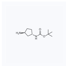
1064788 现货 CAS: 645400-44-8
