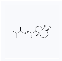
1076016 现货 CAS: 55812-80-1
