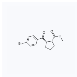
1048755 现货 CAS: 791594-14-4
