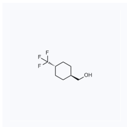
1120268 现货 CAS: 1202577-61-4
