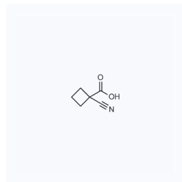
1123225 现货 CAS: 30491-91-9
