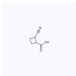
1122557 现货 CAS: 1508446-57-8
