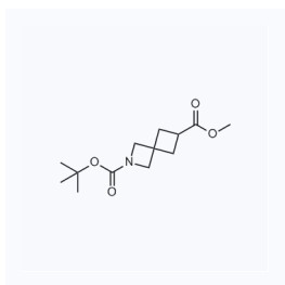
1122436 CAS: 1408074-81-6
