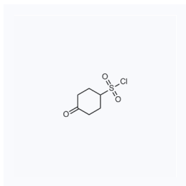
1201060 现货 CAS: 1262409-43-7
