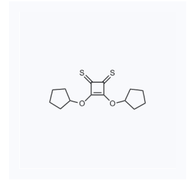
1117213 CAS: 2171494-72-5
