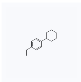
1053384 现货 CAS: 4501-39-7
