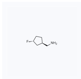
1126457 CAS: 1903832-63-2
