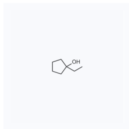
1021714 CAS: 1462-96-0
