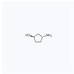
1101221 CAS: 946826-74-0
