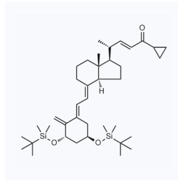
1056975 现货 CAS: 112849-17-9
