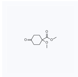
1170713 现货 CAS: 1622928-67-9
