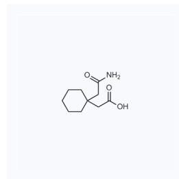
1137857 现货 CAS: 99189-60-3
