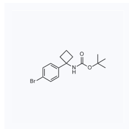
1057510 现货 CAS: 1032350-06-3
