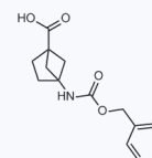
1179560 现货 CAS: 2231674-62-5
