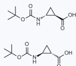
1066681 现货 CAS: 1212381-16-2
