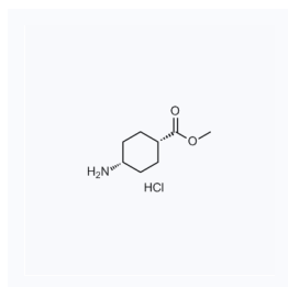
1063591 现货 CAS: 61367-16-6
