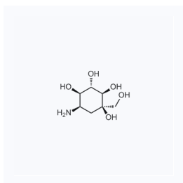
1199249 现货 CAS: 83465-22-9
