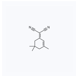
1190726 现货 CAS: 23051-44-7
