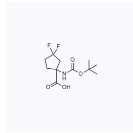
1204763 CAS: 1936649-94-3
