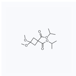
1123413 现货 CAS: 115118-68-8
