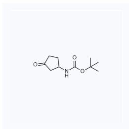
1062424 现货 CAS: 847416-99-3
