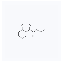
1058494 现货 CAS: 5396-14-5
