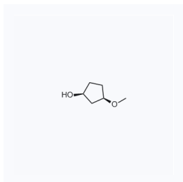
1128632 CAS: 16327-02-9
