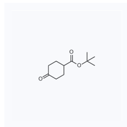
1113775 现货 CAS: 38446-95-6
