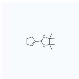
1062219 现货 CAS: 287944-10-9
