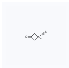
1123087 现货 CAS: 32082-17-0
