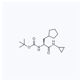
1060551 现货 CAS: 1404457-07-3
