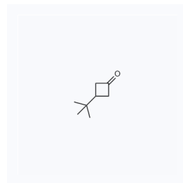
1122417 现货 CAS: 20614-90-8
