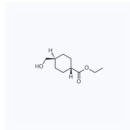
1064513 现货 CAS: 104802-52-0
