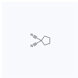
1169203 CAS: 29739-46-6
