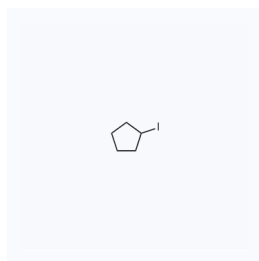
1137790 现货 CAS: 1556-18-9
