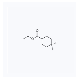
1024016 现货 CAS: 178312-47-5
