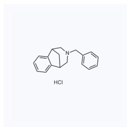
1066848 现货 CAS: 1144040-56-1
