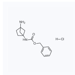
1162634 现货 CAS: 1354951-84-0
