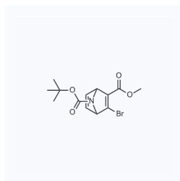
1110267 现货 CAS: 181873-33-6
