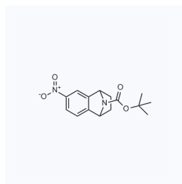
1048455 现货 CAS: 942492-08-2
