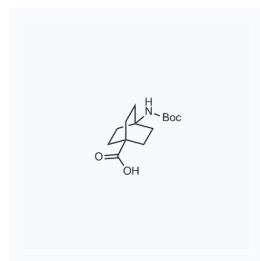
1051019 现货 CAS: 863304-76-1
