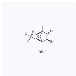
1129111 现货 CAS: 14575-84-9
