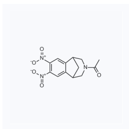
1067318 现货 CAS: 1213782-02-5
