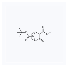
1116931 现货 CAS: 910332-68-2
