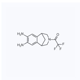
1066814 现货 CAS: 230615-69-7
