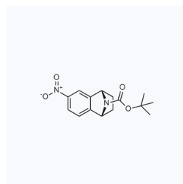
1049217 现货 CAS: 942492-10-6
