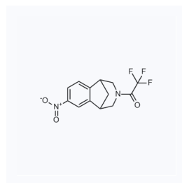
1067003 现货 CAS: 230615-53-9
