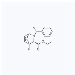
1060324 现货 CAS: 134984-63-7
