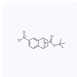
1059098 现货 CAS: 942492-09-3
