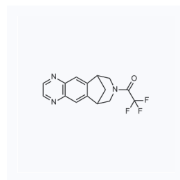
1058201 现货 CAS: 230615-70-0
