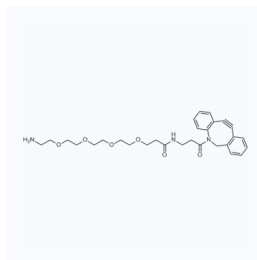
1156986 CAS: 1255942-08-5
