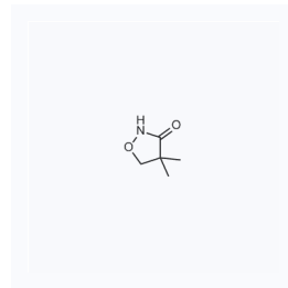
1138515 CAS: 81778-07-6
