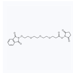
1175679 CAS: 2101206-14-6
