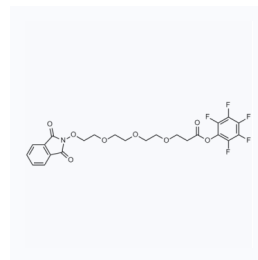
1175678 CAS: 2101206-87-3
