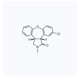
1058632 现货 CAS: 165890-26-6
