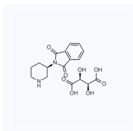
1060376 现货 CAS: 886588-62-1
