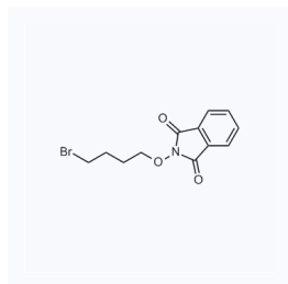
1203120 现货 CAS: 5093-32-3
