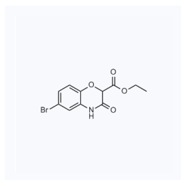
1115219 现货 CAS: 1245708-51-3
