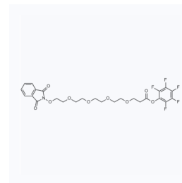
1175642 CAS: 2101206-46-4
