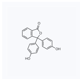
1042729 现货 CAS: 77-09-8
