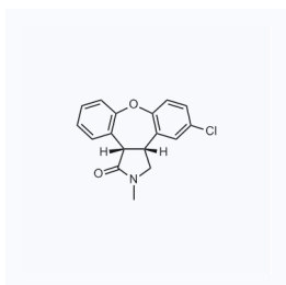
1058245 现货 CAS: 912356-09-3
