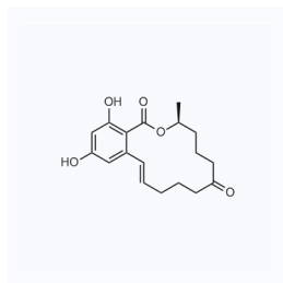
1098986 现货 CAS: 17924-92-4
