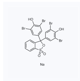
1199021 CAS: 34725-61-6
