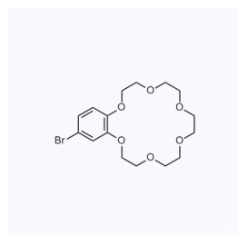
1042040 现货 CAS: 75460-28-5
