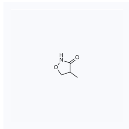
1138875 CAS: 62242-99-3
