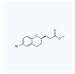
1159854 现货 CAS: 2088284-57-3
