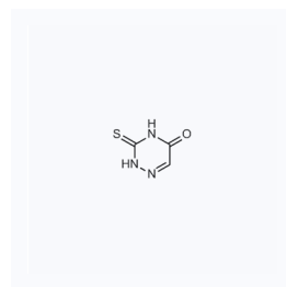
1201043 CAS: 626-08-4
