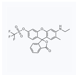
1066997 现货 CAS: 1403936-34-4
