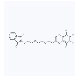
1175681 CAS: 2101206-47-5
