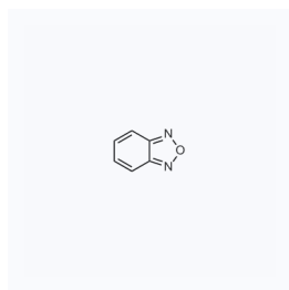
1028052 CAS: 273-09-6
