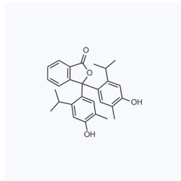
1115248 CAS: 6869-00-7
