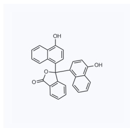
1199381 现货 CAS: 596-01-0
