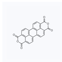
1019262 现货 CAS: 128-69-8
