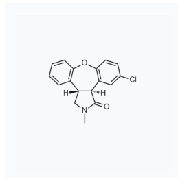
1058631 现货 CAS: 129385-59-7
