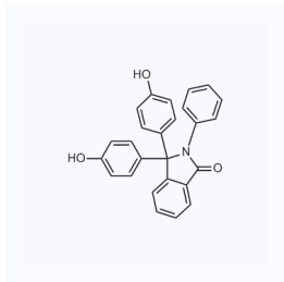
1059254 现货 CAS: 6607-41-6
