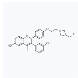
1147778 现货 CAS: 1642297-53-7
