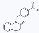
1203126 CAS: 857492-98-9
