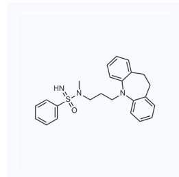
1180410 现货 CAS: 2378147-02-3
