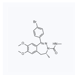
1164705 现货 CAS: 1564271-34-6
