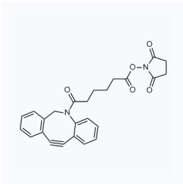
1158012 CAS: 1384870-47-6
