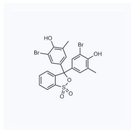
1199399 现货 CAS: 115-40-2
