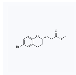
1159855 现货 CAS: 2088284-58-4
