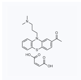
1069330 现货 CAS: 3598-37-6
