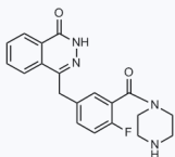
1058771 现货 CAS: 763111-47-3
