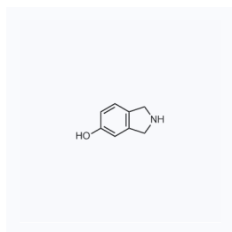
1125647 CAS: 54544-67-1
