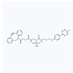
1185108 CAS: 1802238-48-7
