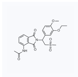
1066756 现货 CAS: 253168-86-4
