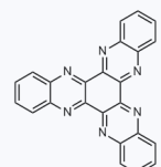
1181708 CAS: 214-83-5
