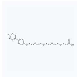
1185566 CAS: 1802907-91-0
