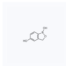
1123381 CAS: 1187190-70-0
