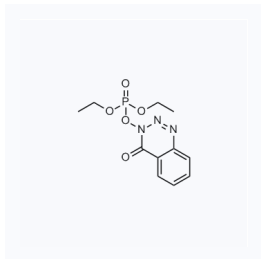
1023138 现货 CAS: 165534-43-0
