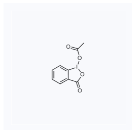
1051231 现货 CAS: 1829-26-1
