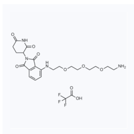
1170906 现货 CAS: 2414913-97-4
