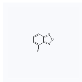
1028553 CAS: 29270-55-1
