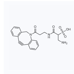
1163155 CAS: 2028284-70-8
