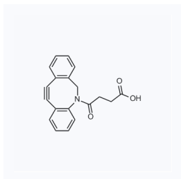
1115016 现货 CAS: 1353016-70-2
