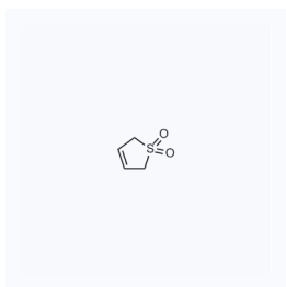
1141691 CAS: 77-79-2
