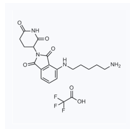
1170088 现货 CAS: 2093386-40-2
