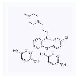
1044534 现货 CAS: 84-02-6
