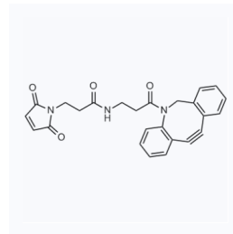
1135224 CAS: 1395786-30-7
