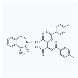
1057528 现货 CAS: 425386-58-9
