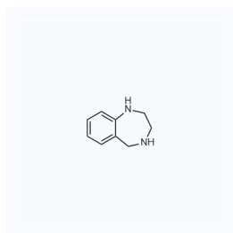
1197386 CAS: 5946-39-4
