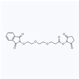
1175682 CAS: 2101206-31-7
