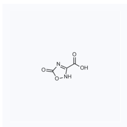
1139538 CAS: 1257265-24-9
