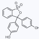
1080107 现货 CAS: 143-74-8
