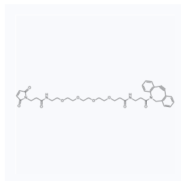
1149761 CAS: 1480516-75-3
