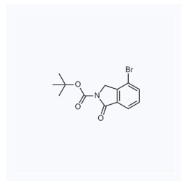
1201826 现货 CAS: 658683-18-2
