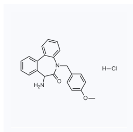
1060620 现货 CAS: 1083065-04-6
