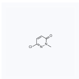
1147393 CAS: 10071-38-2
