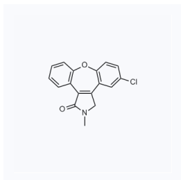
1058243 现货 CAS: 934996-79-9
