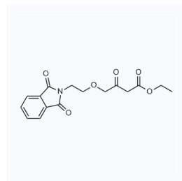
1132253 现货 CAS: 88150-75-8
