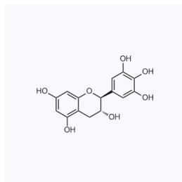
1030010 现货 CAS: 3371-27-5
