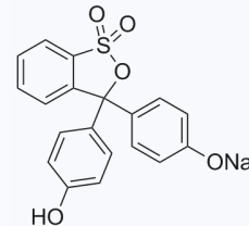
1080108 现货 CAS: 34487-61-1
