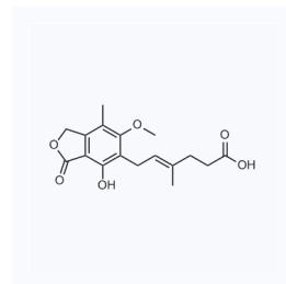
1026973 现货 CAS: 24280-93-1
