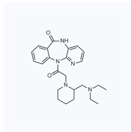
1015186 CAS: 102394-31-0
