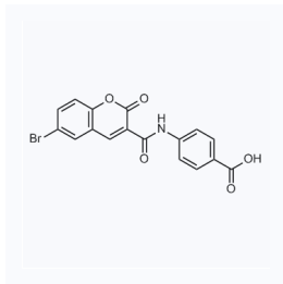
1143454 CAS: 312756-47-1
