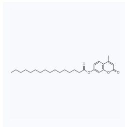
1023931 CAS: 17695-48-6
