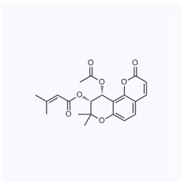
1033340 CAS: 477-33-8
