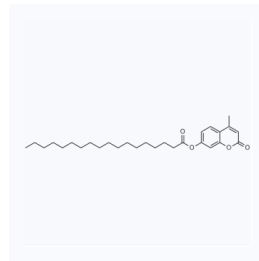
1092481 CAS: 79408-85-8
