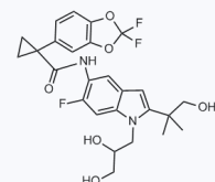
1079126 CAS: 1226709-85-8
