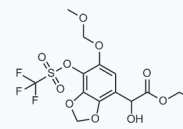
1060578 CAS: 874758-54-0
