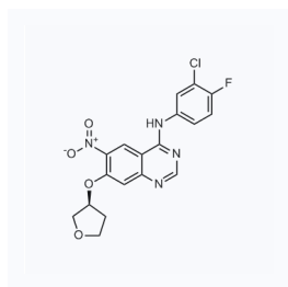
1057257 现货 CAS: 314771-88-5
