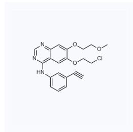
1059685 现货 CAS: 183321-83-7
