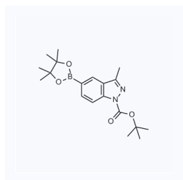
1156007 现货 CAS: 864770-82-1
