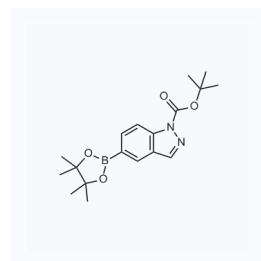
1069952 现货 CAS: 864771-44-8
