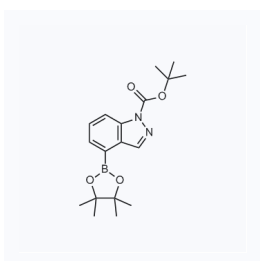
1126816 CAS: 1446443-06-6
