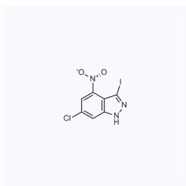
1174131 现货 CAS: 885519-97-1
