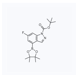
1124968 CAS: 1333319-72-4
