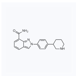
1079909 现货 CAS: 1038915-75-1
