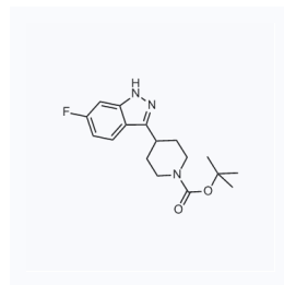
1051522 CAS: 1198284-41-1
