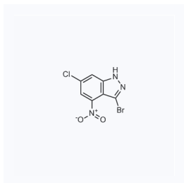
1111853 现货 CAS: 885519-92-6
