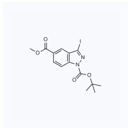
1172291 现货 CAS: 944904-57-8
