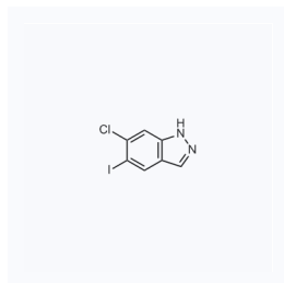
1106760 现货 CAS: 1227269-39-7
