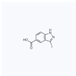
1111785 现货 CAS: 885521-46-0
