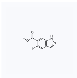
1167104 现货 CAS: 1227268-85-0
