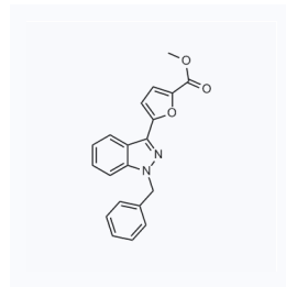
1049489 CAS: 170632-13-0
