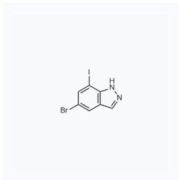
1190405 CAS: 953410-86-1
