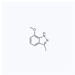
1111877 现货 CAS: 351210-07-6
