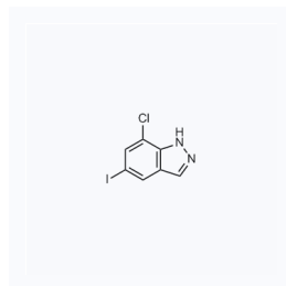
1201683 现货 CAS: 1000343-56-5
