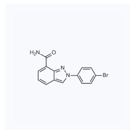
1106057 现货 CAS: 952478-17-0
