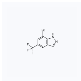
1111952 现货 CAS: 1100212-66-5
