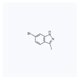
1120915 现货 CAS: 885521-88-0
