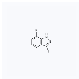
1120668 现货 CAS: 944904-38-5
