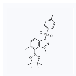
1124965 CAS: 1421252-90-5
