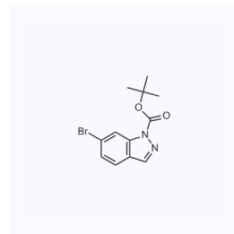
1064440 现货 CAS: 877264-77-2
