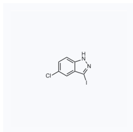
1069068 现货 CAS: 351456-45-6
