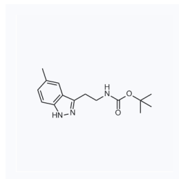
1105703 现货 CAS: 1956370-87-8
