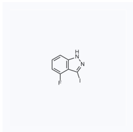
1064644 现货 CAS: 518990-32-4
