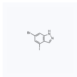
1111651 现货 CAS: 885519-41-5
