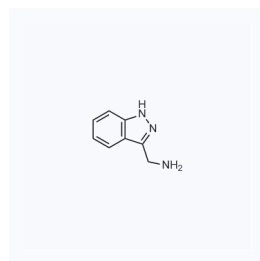
1052456 现货 CAS: 806640-37-9
