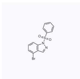
1123481 CAS: 1001415-32-2
