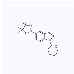
1059290 CAS: 1082525-64-1
