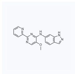
1050022 CAS: 1447606-32-7
