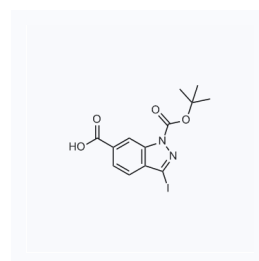
1050085 CAS: 1799420-87-3
