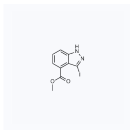
1119726 现货 CAS: 885521-54-0
