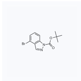
1052918 现货 CAS: 926922-37-4
