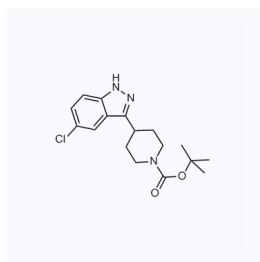
1051073 CAS: 1198284-74-0
