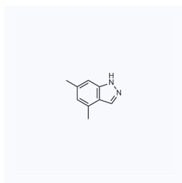
1124953 现货 CAS: 43120-31-6
