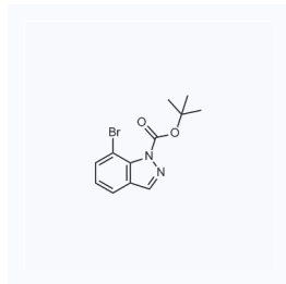
1076118 现货 CAS: 1092352-37-8
