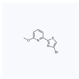
1059090 现货 CAS: 1415559-65-7
