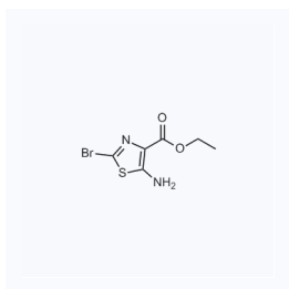
1166787 现货 CAS: 1228281-54-6
