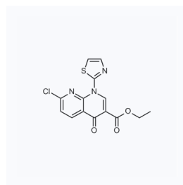
1060012 现货 CAS: 174726-87-5
