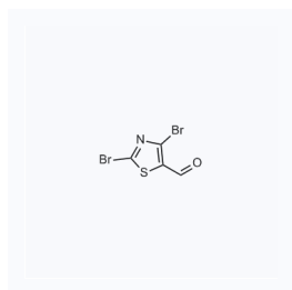
1068060 现货 CAS: 139669-95-7
