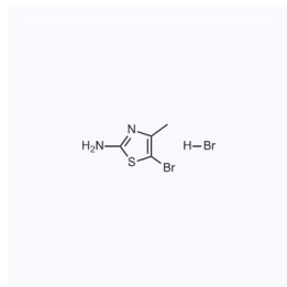
1171305 现货 CAS: 79247-77-1
