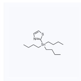
1111605 现货 CAS: 121359-48-6
