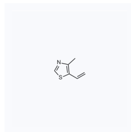
1023869 现货 CAS: 1759-28-0
