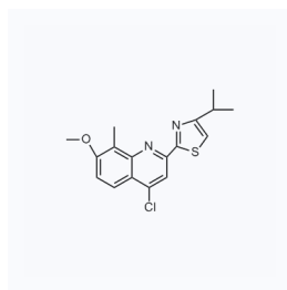
1057028 现货 CAS: 1193272-59-1
