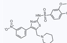
1014848 CAS: 1008119-83-2
