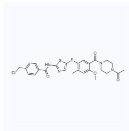
1057330 CAS: 439578-99-1
