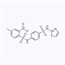
1207872 现货 CAS: 712326-63-1
