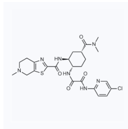
1126351 CAS: 1255529-28-2
