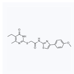
1035648 现货 CAS: 552309-42-9
