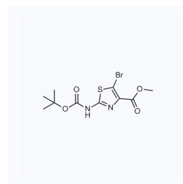
1114313 现货 CAS: 914349-71-6
