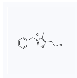
1033018 现货 CAS: 4568-71-2
