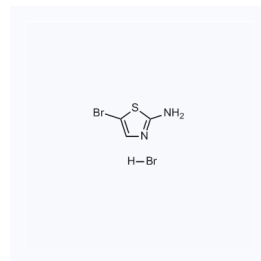
1037680 现货 CAS: 61296-22-8
