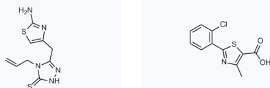
1141990 CAS: 690643-10-8
