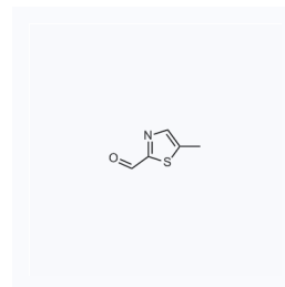
1052578 现货 CAS: 13838-78-3
