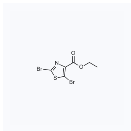
1067411 现货 CAS: 208264-60-2
