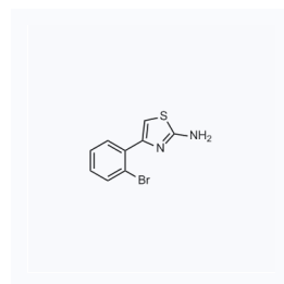
1176840 现货 CAS: 103965-99-7
