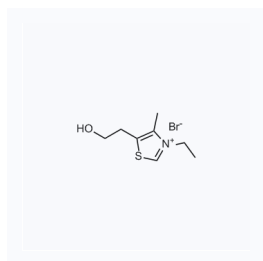
1035158 现货 CAS: 54016-70-5
