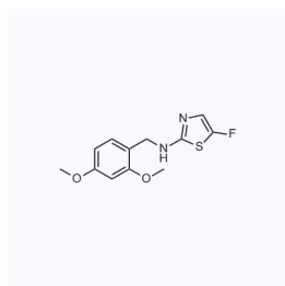
1110163 现货 CAS: 2007920-92-3
