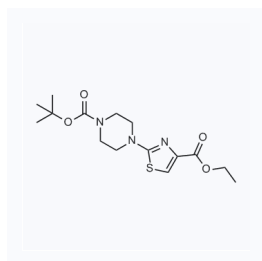
1089046 现货 CAS: 867065-53-0
