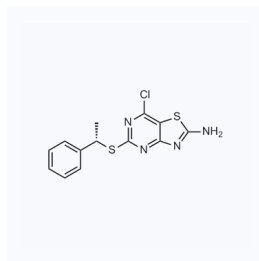
1066768 现货 CAS: 911820-08-1
