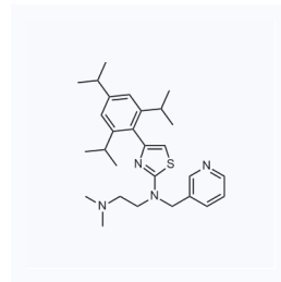
1020568 现货 CAS: 136468-36-5
