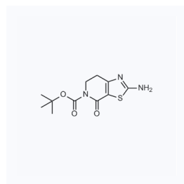
1166479 现货 CAS: 1312412-88-6
