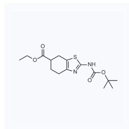
1166603 现货 CAS: 1820647-12-8
