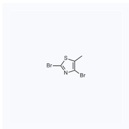
1063397 现货 CAS: 1206708-88-4
