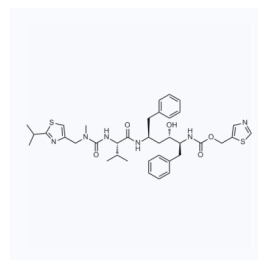
1022474 现货 CAS: 155213-67-5
