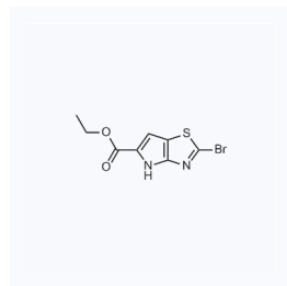
1114804 现货 CAS: 1379315-43-1
