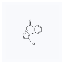
1068717 现货 CAS: 341028-37-3
