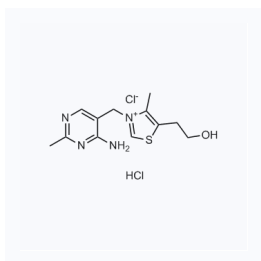
1039494 现货 CAS: 67-03-8
