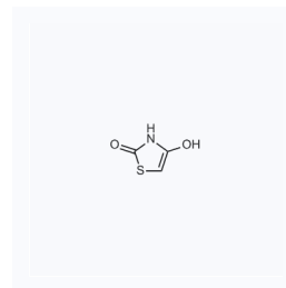
1137983 现货 CAS: 625-85-4
