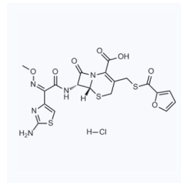
1015500 CAS: 103980-44-5
