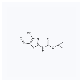
1111025 现货 CAS: 944805-17-8
