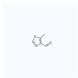
1125617 现货 CAS: 261710-79-6
