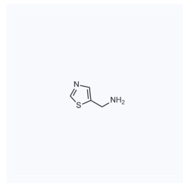
1063695 现货 CAS: 161805-76-1
