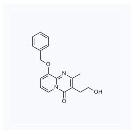
1058573 现货 CAS: 1008796-22-2
