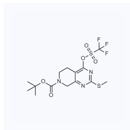
1166329 现货 CAS: 338739-82-5
