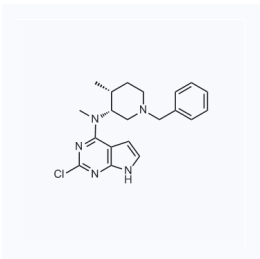
1059247 现货 CAS: 923036-25-3
