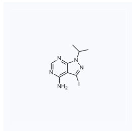
1066241 现货 CAS: 862730-04-9
