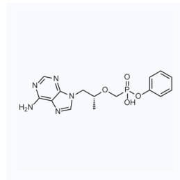
1091913 现货 CAS: 379270-35-6
