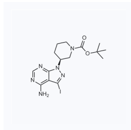
1112927 现货 CAS: 461702-66-9
