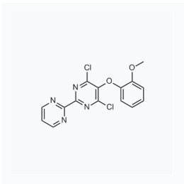
1022135 现货 CAS: 150728-13-5
