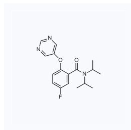
1169861 现货 CAS: 2169919-95-1
