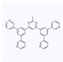
1133413 现货 CAS: 925425-96-3
