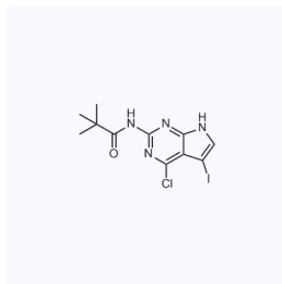
1069935 现货 CAS: 149765-16-2
