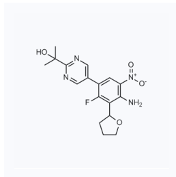
1127468 现货 CAS: 1384984-28-4
