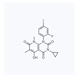
1058808 现货 CAS: 871700-24-2
