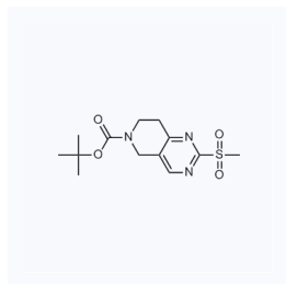
1052793 现货 CAS: 259809-79-5
