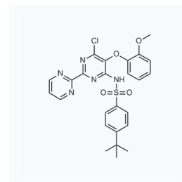
1058164 现货 CAS: 150727-06-3
