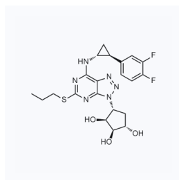
1060061 现货 CAS: 220347-05-7
