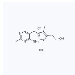
1039494 现货 CAS: 67-03-8
