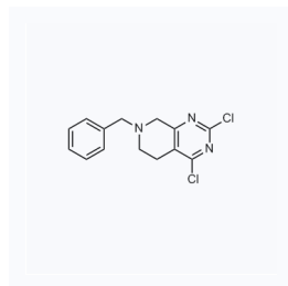
1059689 现货 CAS: 1059735-34-0
