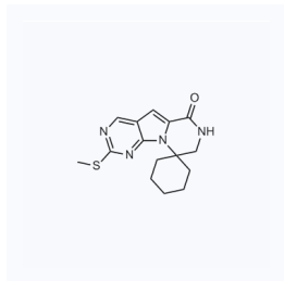
1135367 现货 CAS: 2170747-00-7
