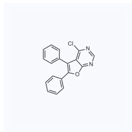
1059894 现货 CAS: 65148-07-4
