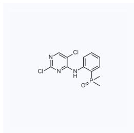
1099242 现货 CAS: 1197953-49-3
