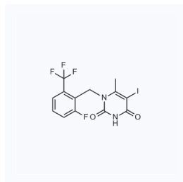
1123304 现货 CAS: 1150560-54-5
