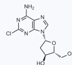
1032575 现货 CAS: 4291-63-8
