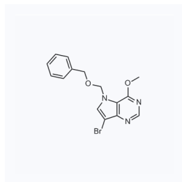
1061261 现货 CAS: 299916-62-4
