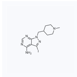
1112928 现货 CAS: 1411763-96-6
