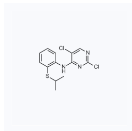
1060529 现货 CAS: 1632485-14-3
