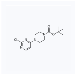
1052230 现货 CAS: 221050-88-0
