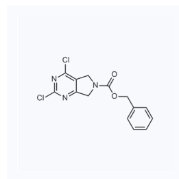
1170763 现货 CAS: 1990514-48-1
