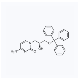
1060162 现货 CAS: 132336-30-2
