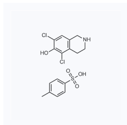
1114879 现货 CAS: 1609545-55-2
