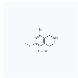
1203185 CAS: 2411640-34-9
