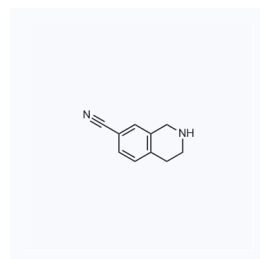
1166883 CAS: 149355-52-2
