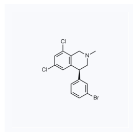
1066766 现货 CAS: 1870821-29-6
