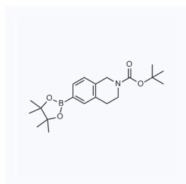
1105943 现货 CAS: 893566-72-8
