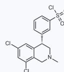
1101713 CAS: 1610028-57-3
