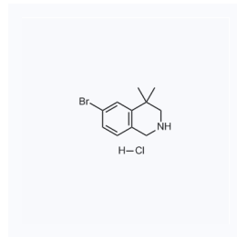
1206924 CAS: 1203684-61-0
