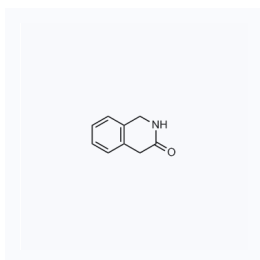
1190665 CAS: 24331-94-0
