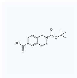
1063580 CAS: 170097-67-3
