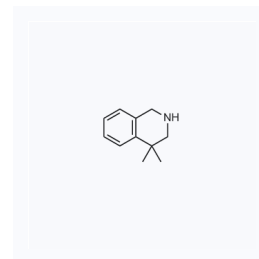
1141676 CAS: 78592-91-3
