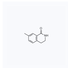
1143148 CAS: 371756-25-1
