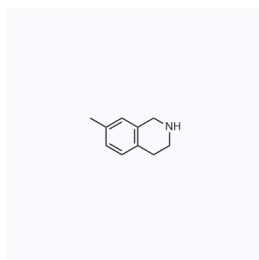
1069310 CAS: 207451-81-8
