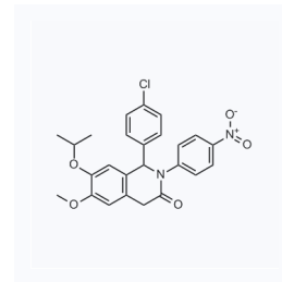
1060587 现货 CAS: 1821463-86-8
