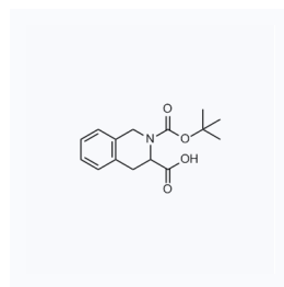
1111285 CAS: 151838-62-9
