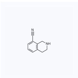
1126878 CAS: 215798-85-9
