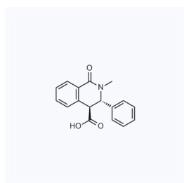
1142326 CAS: 60734-32-9
