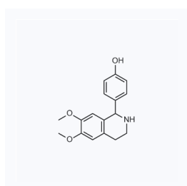
1143511 CAS: 301325-93-9
