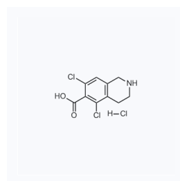
1200500 CAS: 1289646-93-0
