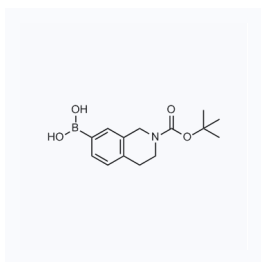
1160638 CAS: 1190058-21-9
