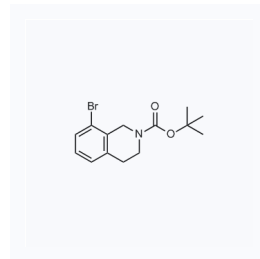
1064908 现货 CAS: 893566-75-1
