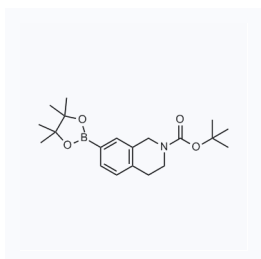
1050374 现货 CAS: 937048-76-5
