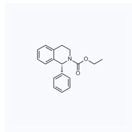
1058458 现货 CAS: 180468-41-1
