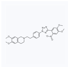
1150078 现货 CAS: 849675-45-2
