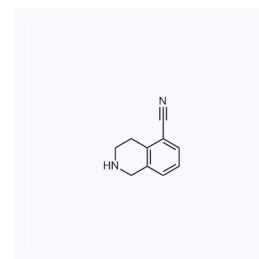
1129200 CAS: 215794-24-4
