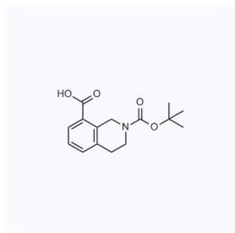
1061864 现货 CAS: 878798-87-9
