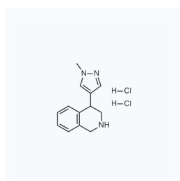
1149610 CAS: 1949816-17-4
