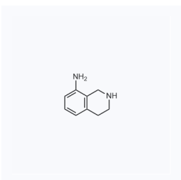
1067789 CAS: 924633-49-8
