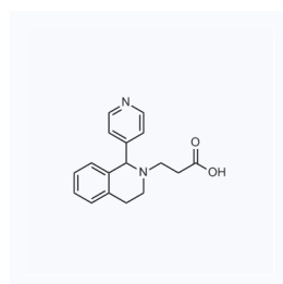
1142313 CAS: 610258-80-5
