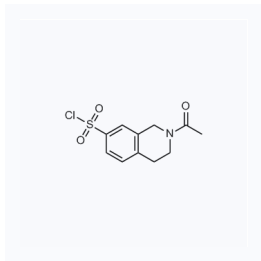
1142264 CAS: 61563-39-1
