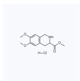
1190684 CAS: 30740-96-6
