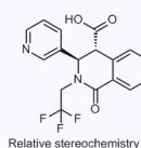
1105563 CAS: 1424799-69-8
