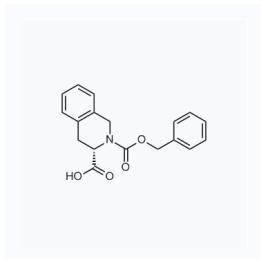
1051985 现货 CAS: 79261-58-8
