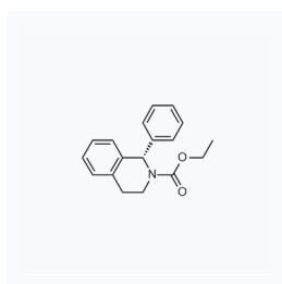
1057986 CAS: 180468-42-2
