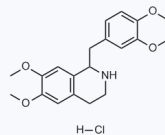
1038946 CAS: 6429-04-5
