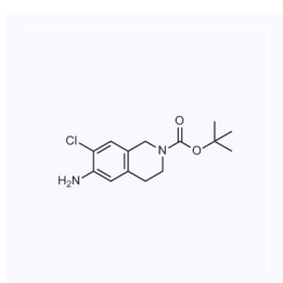
1172704 CAS: 912846-75-4
