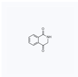
1132857 CAS: 31053-30-2
