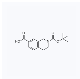
1063964 现货 CAS: 149353-95-7
