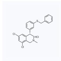
1092640 现货 CAS: 2322360-87-0
