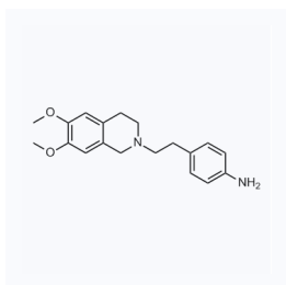
1044400 现货 CAS: 82925-02-8
