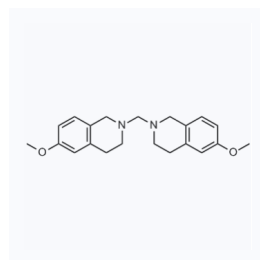
1061219 现货 CAS: 942150-85-8
