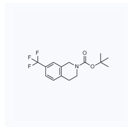
1111732 现货 CAS: 1257855-77-8
