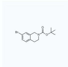
1062949 现货 CAS: 258515-65-0
