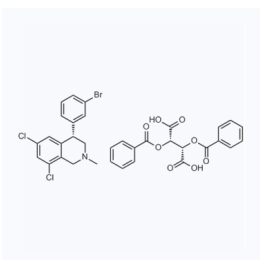
1066715 现货 CAS: 1870821-30-9
