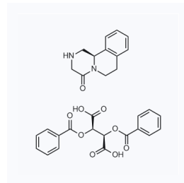
1061902 现货 CAS: 1399880-37-5
