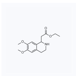
1132259 CAS: 14028-68-3
