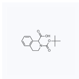
1052615 CAS: 166591-85-1
