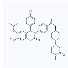
1060590 现货 CAS: 1313363-86-8
