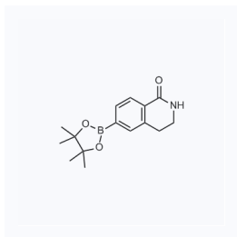
1133125 CAS: 376584-30-4
