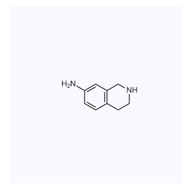
1115129 CAS: 72299-68-4
