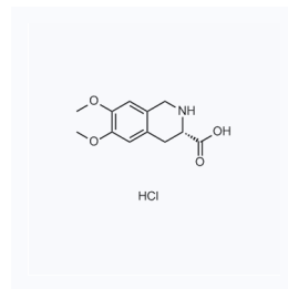
1105708 CAS: 82586-62-7
