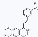
1141448 CAS: 865546-41-4
