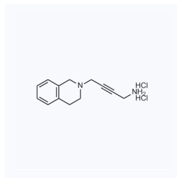
1145416 CAS: 1396785-03-7
