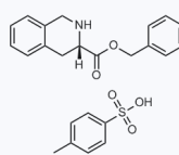
1042859 CAS: 77497-97-3
