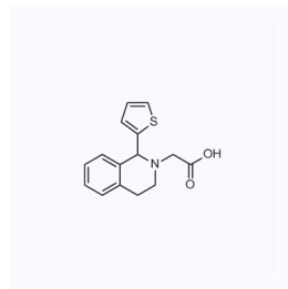
1141391 CAS: 872696-23-6
