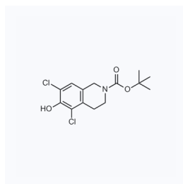
1114880 现货 CAS: 851784-76-4
