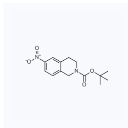
1049043 现货 CAS: 186390-79-4
