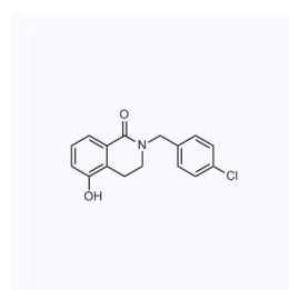
1146738 CAS: 1105196-16-4
