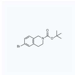
1065813 现货 CAS: 893566-74-0
