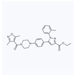
1058120 CAS: 1007477-05-5
