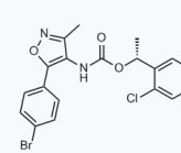
1059425 CAS: 1228690-20-7
