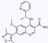
1059773 CAS: 1300737-69-2
