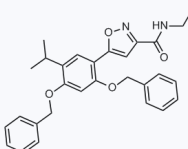
1057545 CAS: 747414-21-7
