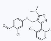
1058751 CAS: 278597-32-3
