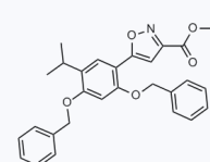
1057548 CAS: 747414-20-6
