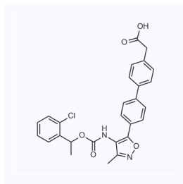
1059455 CAS: 1228689-85-7
