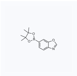
1203142 现货 CAS: 1810038-58-4
