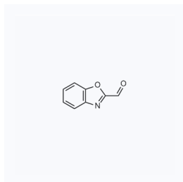
1069346 现货 CAS: 62667-25-8
