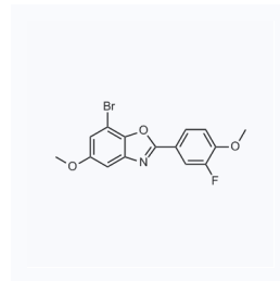
1061545 CAS: 544704-75-8
