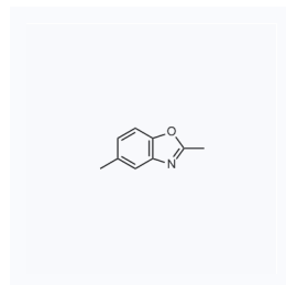
1036150 现货 CAS: 5676-58-4
