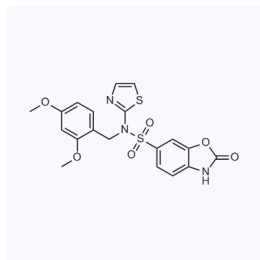
1105730 现货 CAS: 1432515-21-3
