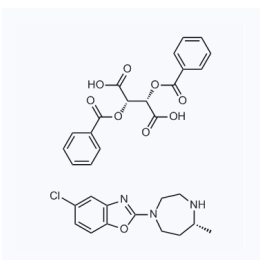
1057648 CAS: 1276666-14-8
