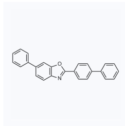
1023496 CAS: 17064-47-0
