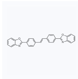
1022354 CAS: 1533-45-5
