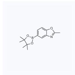
1166665 现货 CAS: 845872-30-2
