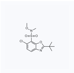
1050434 CAS: 1206896-20-9
