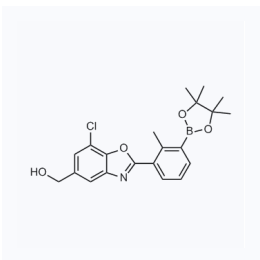
1179724 现货 CAS: 2230904-26-2
