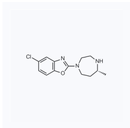
1049159 现货 CAS: 1266975-27-2
