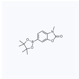
1064286 现货 CAS: 1016641-53-4
