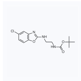
1049158 现货 CAS: 1144509-75-0
