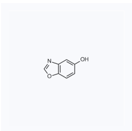
1048054 现货 CAS: 180716-28-3
