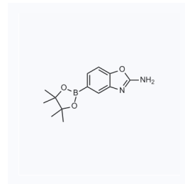
1066338 现货 CAS: 1224844-66-9
