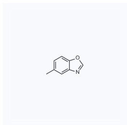
1201084 现货 CAS: 10531-78-9
