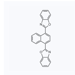
1034098 CAS: 5089-22-5
