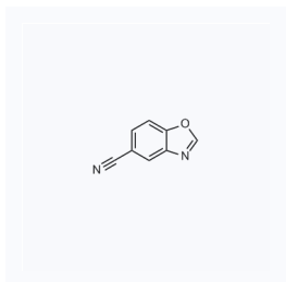
1114760 现货 CAS: 132227-01-1
