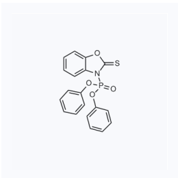
1016833 CAS: 111160-56-6
