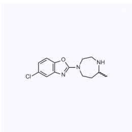
1059131 现货 CAS: 1276666-13-7
