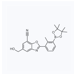
1174476 CAS: 2230904-54-6
