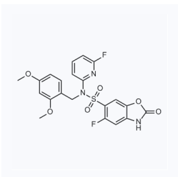
1115272 现货 CAS: 1607485-79-9
