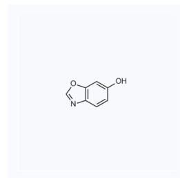
1048089 现货 CAS: 106050-81-1
