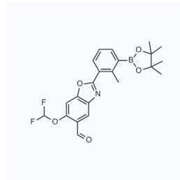
1198860
