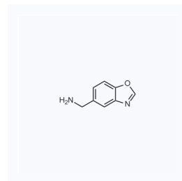
1115371 现货 CAS: 903556-78-5
